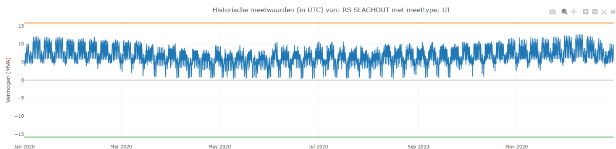
Figuur 3: Gerealiseerde vermogenscurve in het afgelopen jaar bij verdeelstation Slaghout.
