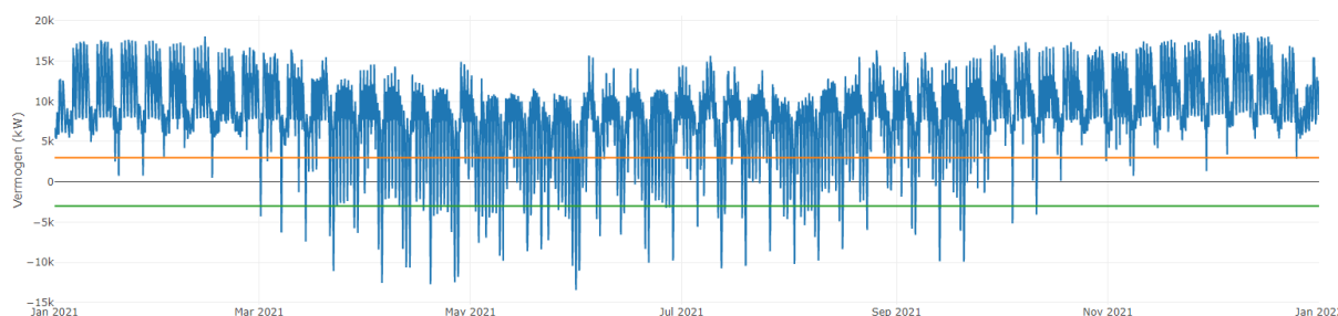
Figuur 4: Verwachte belasting in het laatste jaar van de verwachte congestie bij verdeelstation Slaghout.
