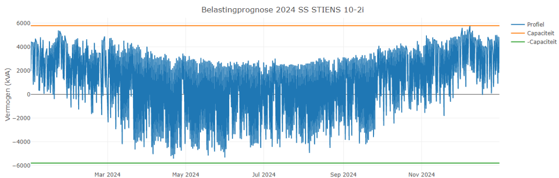
Figuur 4: Verwachte belasting in het laatste jaar van de verwachte congestie bij verdeelstation Stiens .
