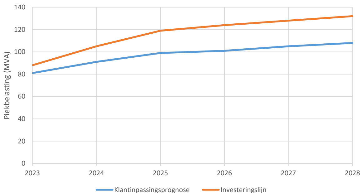
Figuur 4: Verwachte piekbelasting op verdeelstation Zuiderveld per jaar tot en met eind 2028.
