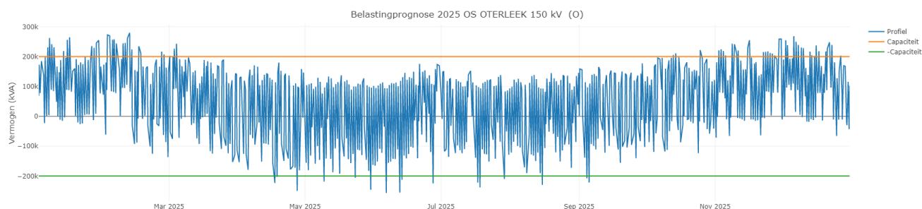
Figuur 7: Verwachte belasting in het laatste jaar van de verwachte congestie bij verdeelstation Oterleek.
