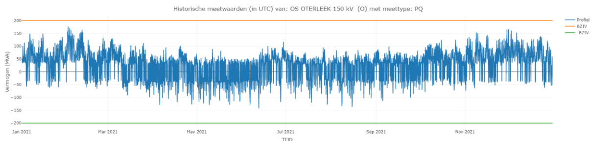
Figuur 6: Gerealiseerde vermogenscurve in het afgelopen jaar bij verdeelstation Oterleek.
