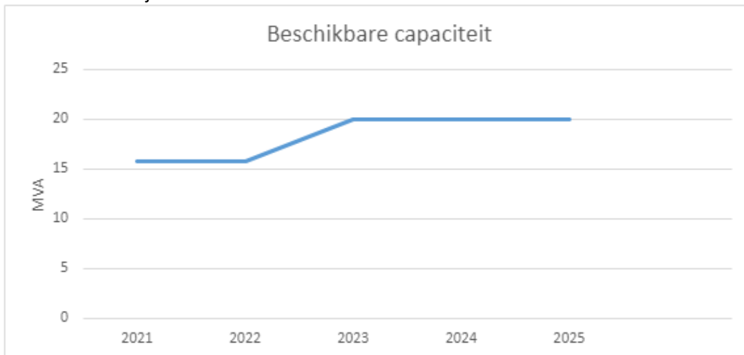
Figuur 3: Ontwikkeling van aanwezige transportcapaciteit in het congestiegebied.
