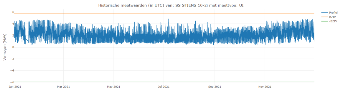
Figuur 4: Gerealiseerde vermogenscurve in het afgelopen jaar bij verdeelstation Stiens .
