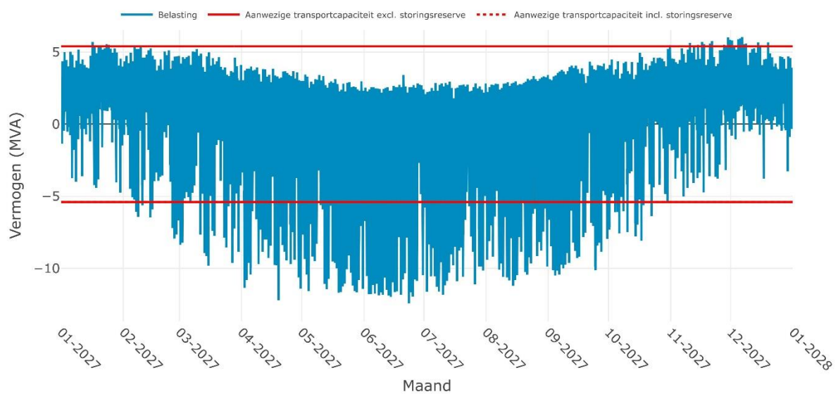
Verwachte belasting op SS STIENS 10-2i voor het jaar 2027
