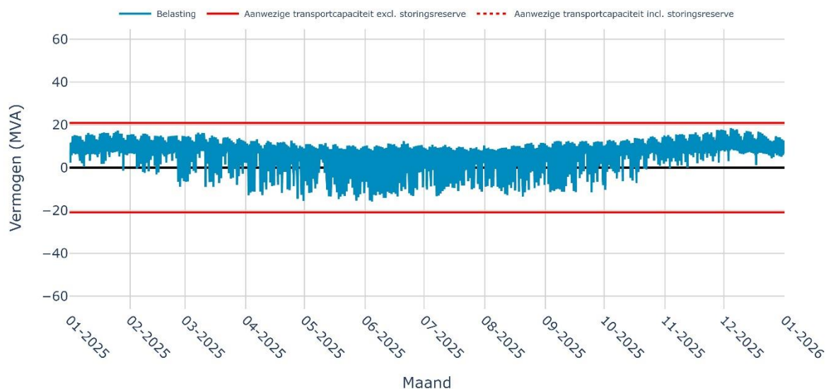
Verwachte belasting op RS HOGE ENK 10-1i + 10-2i voor het jaar 2025
