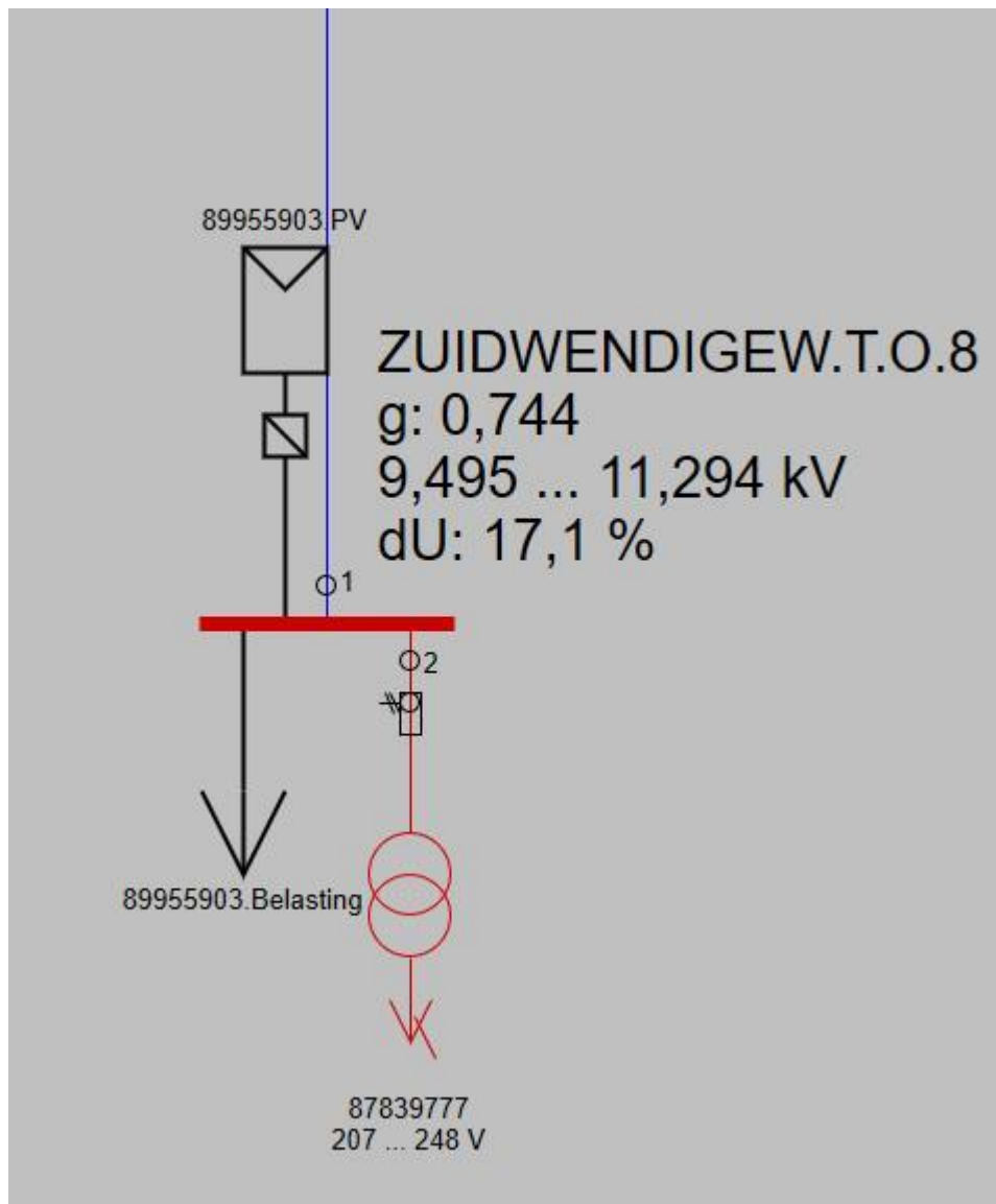
Bijlage: Locatie met slechtste spanningsresultaten welke buiten de beleidsgrenzen vallen Hoge Enk
