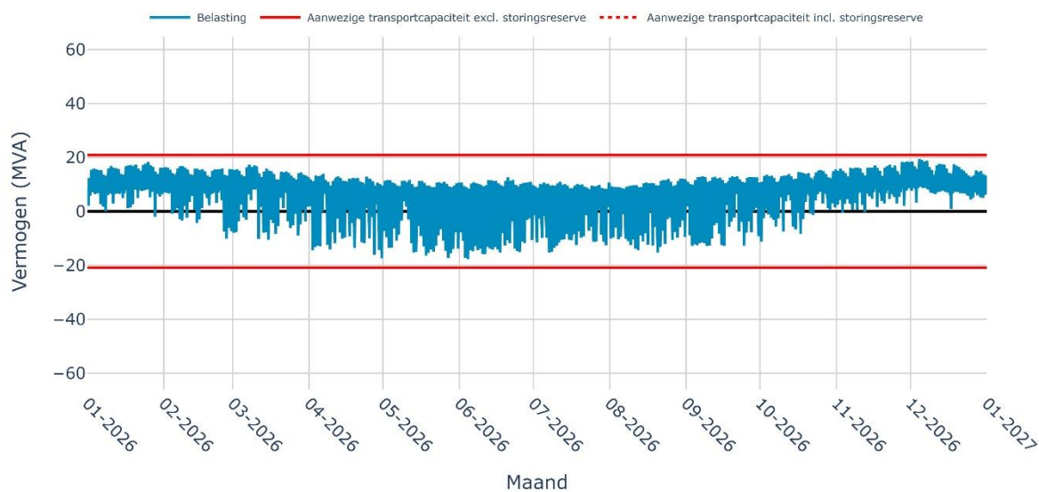
Verwachte belasting op RS HOGE ENK 10-1i + 10-2i voor het jaar 2026
