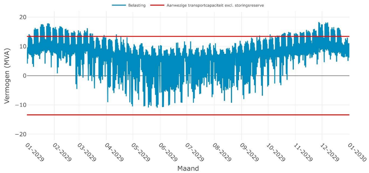
Verwachte belasting op SS HEERENVEEN PIM MULIER 10-1i voor het jaar 2029
