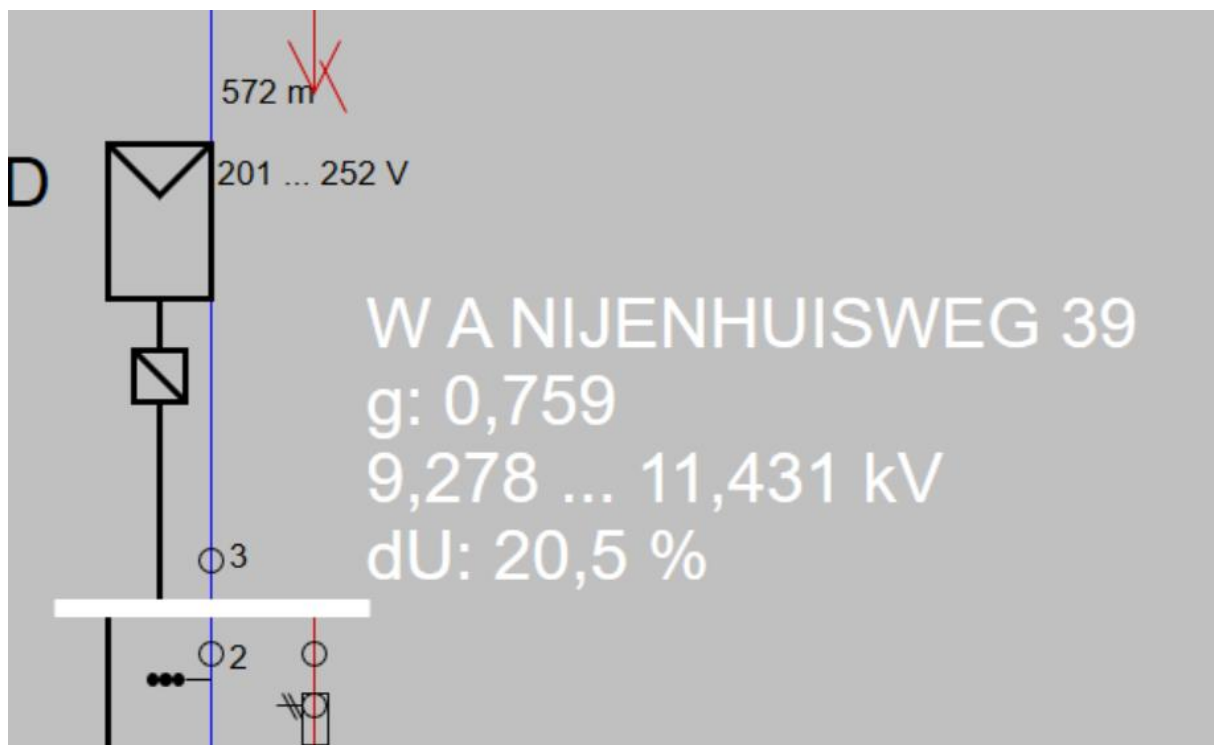
Figuur 3: Locatie met slechtste spanningsresultaten welke buiten de beleidsgrenzen vallen
