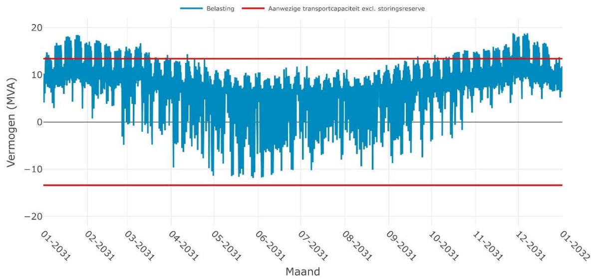
Verwachte belasting op SS HEERENVEEN PIM MULIER 10-1i voor het jaar 2031
