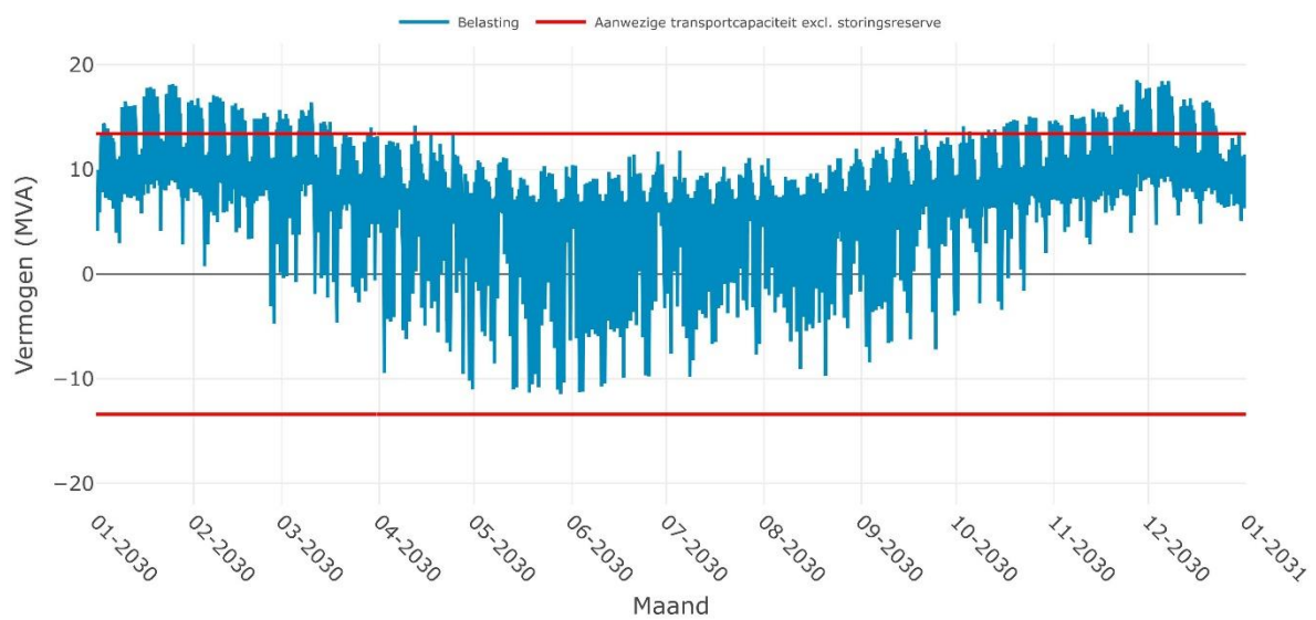
Verwachte belasting op SS HEERENVEEN PIM MULIER 10-1i voor het jaar 2030
