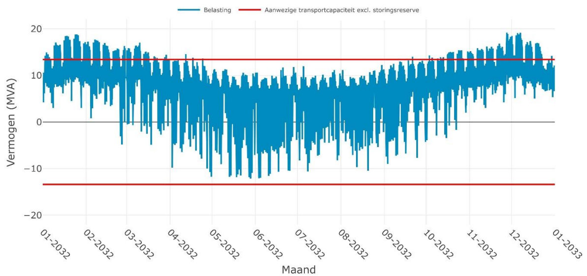
Verwachte belasting op SS HEERENVEEN PIM MULIER 10-1i voor het jaar 2032
