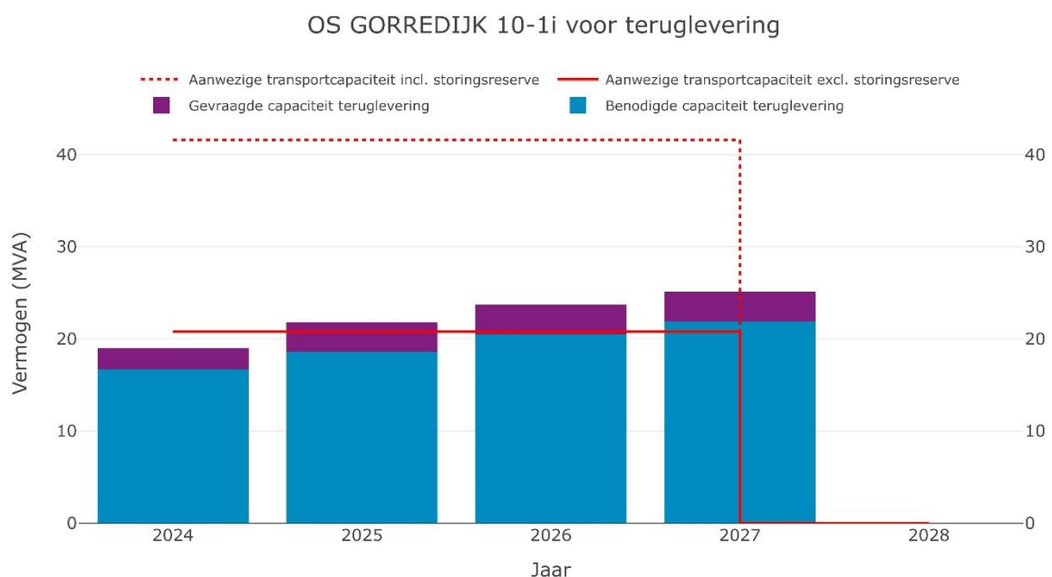
Figuur 2: Ontwikkeling van de aanwezig transportcapaciteit op Congestiegebied Gorredijk tot en met het tweede kwartaal van 2035
