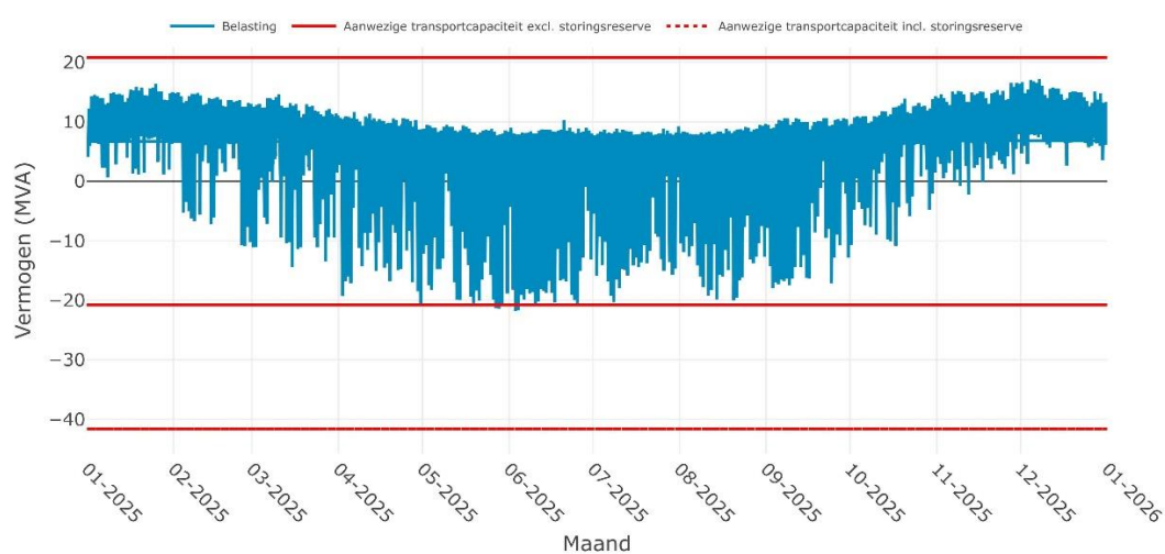
Verwachte belasting op OS GORREDIJK 10-1i voor het jaar 2025
