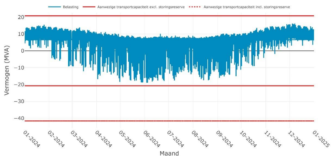
Verwachte belasting op OS GORREDIJK 10-1i voor het jaar 2024
