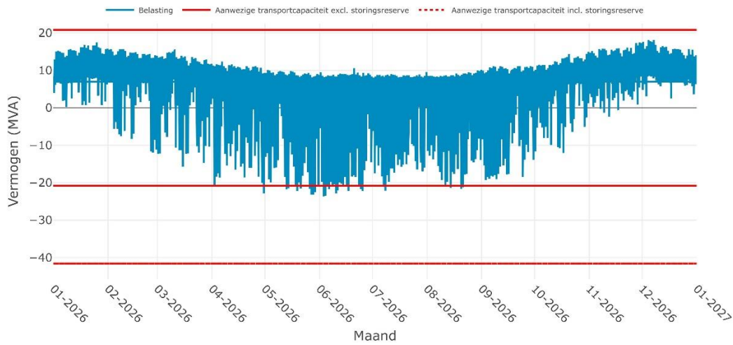
Verwachte belasting op OS GORREDIJK 10-1i voor het jaar 2027
