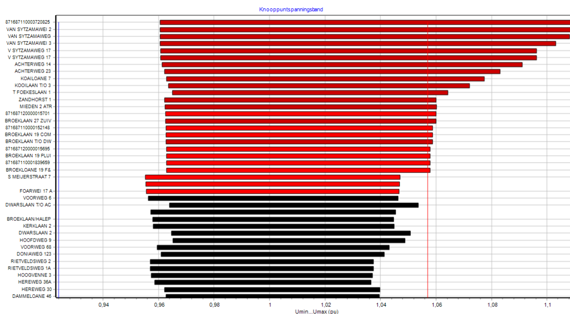
Figuur 2: Spanningscongestie
