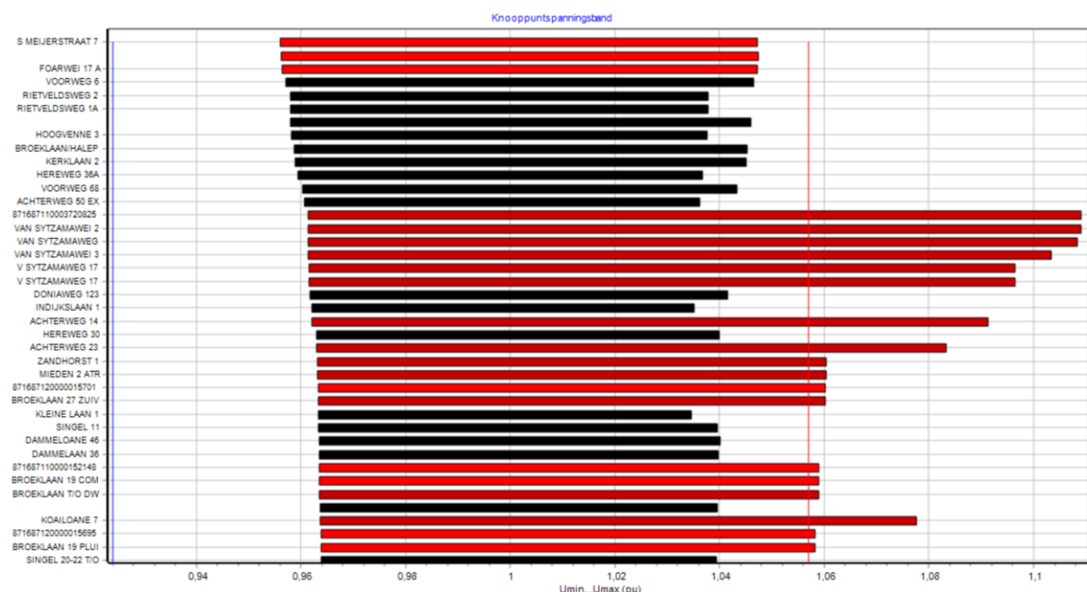
Figuur 2: Spanningscongestie
