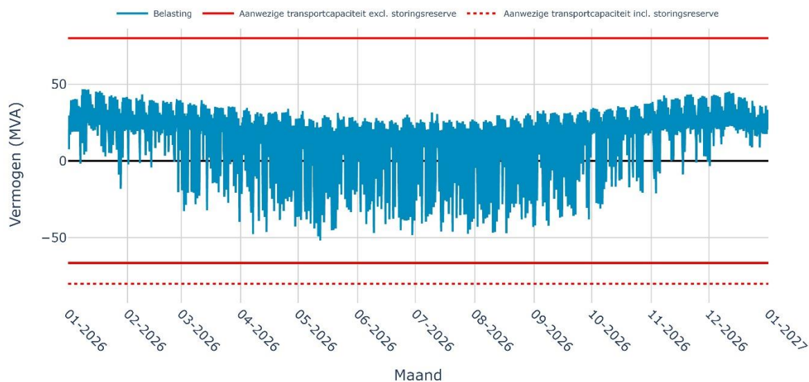
Verwachte belasting op RS BARNEVELD 20-5i voor het jaar 2026
