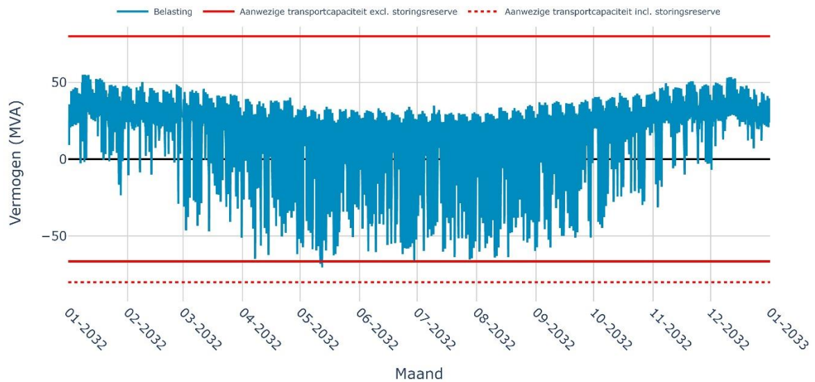
Verwachte belasting op RS BARNEVELD 20-5i voor het jaar 2032
