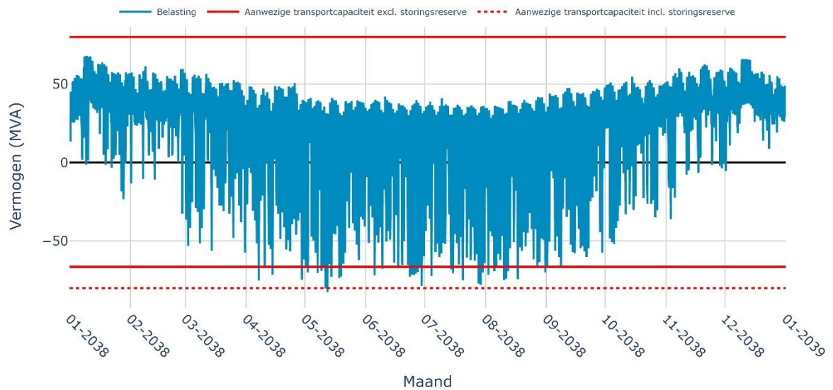
Verwachte belasting op RS BARNEVELD 20-5i voor het jaar 2038
