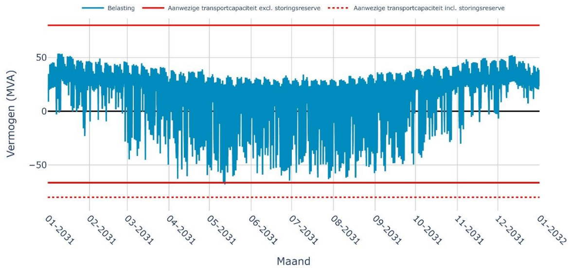
Verwachte belasting op RS BARNEVELD 20-5i voor het jaar 2031
