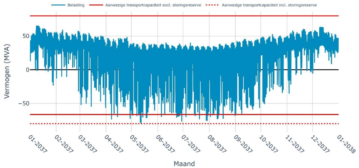
Verwachte belasting op RS BARNEVELD 20-5i voor het jaar 2037
