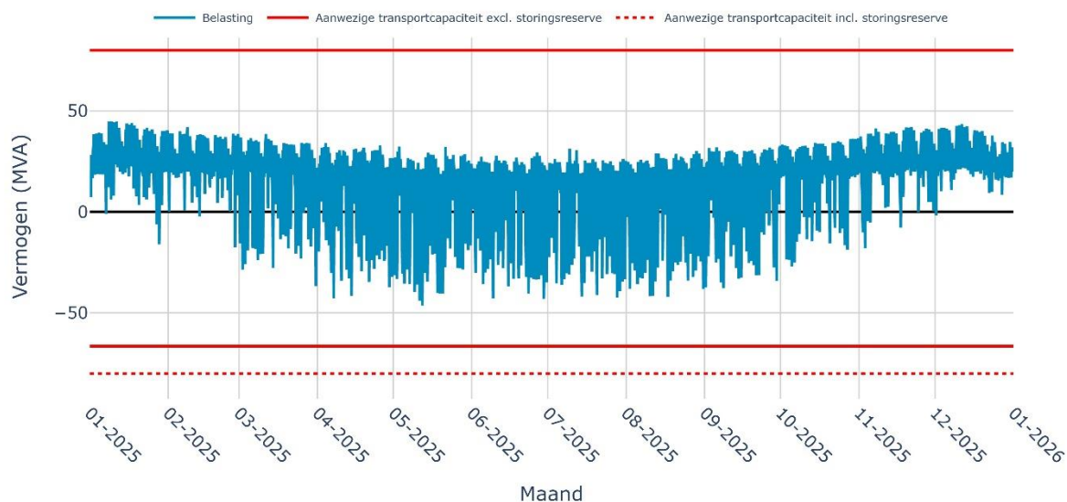
Verwachte belasting op RS BARNEVELD 20-5i voor het jaar 2025
