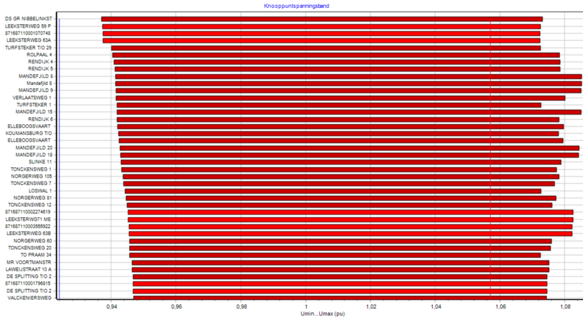
Figuur 2: Spanningscongestie
