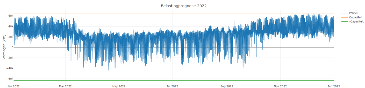
Figuur 7: Verwachte belasting in het laatste jaar van de verwachte congestie bij verdeelstation OS Zaltbommel 10kV installatie I.
