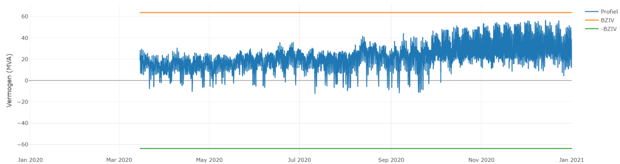
Figuur 6: Gerealiseerde vermogenscurve in het afgelopen jaar bij verdeelstation OS Zaltbommel 10kV installatie I
