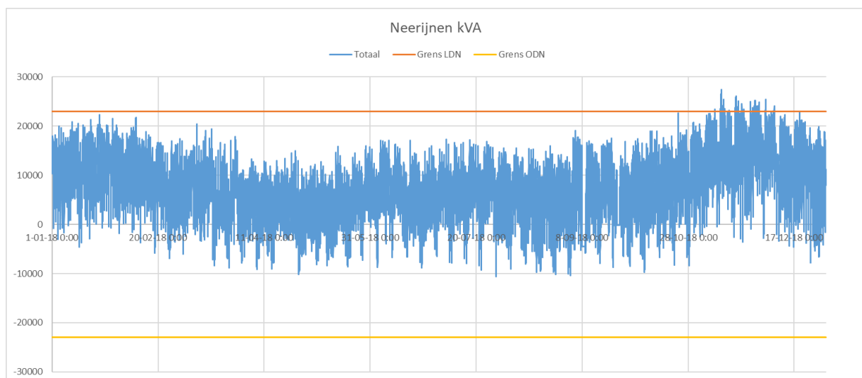
Figuur 7: Gerealiseerde vermogenscurve in 2018 bij verdeelstation Neerijnen.
