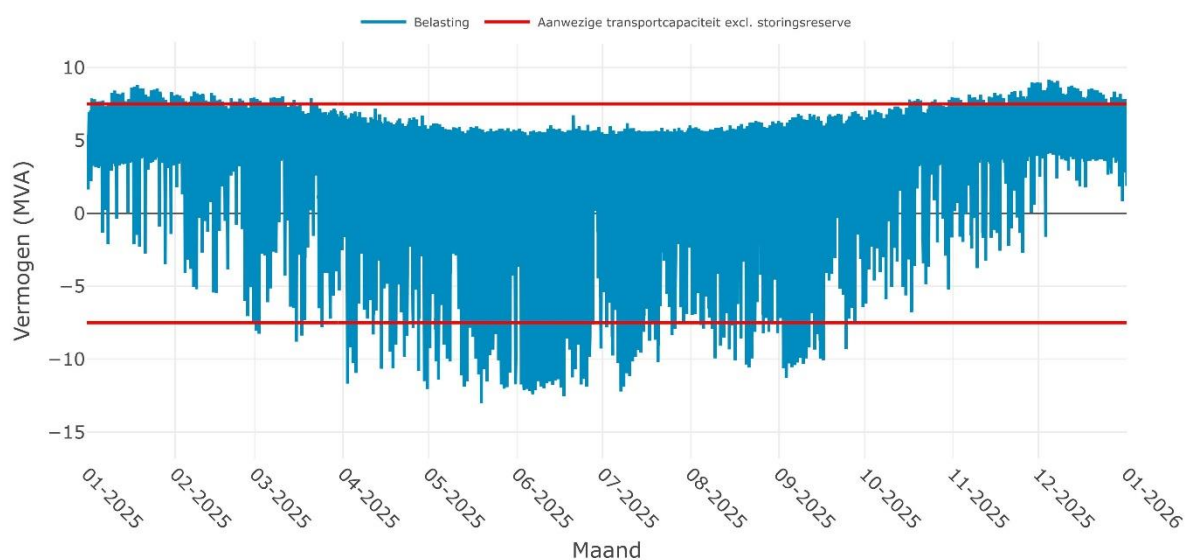
Verwachte belasting op RS WASKEMEER 10-2i voor het jaar 2025
