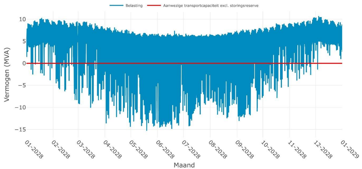
Verwachte belasting op RS WASKEMEER 10-2i voor het jaar 2028
