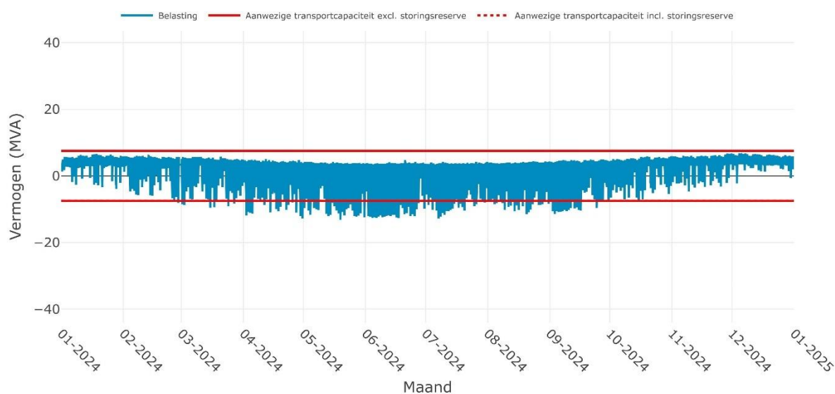
Verwachte belasting op RS WASKEMEER 10-2i voor het jaar 2024
