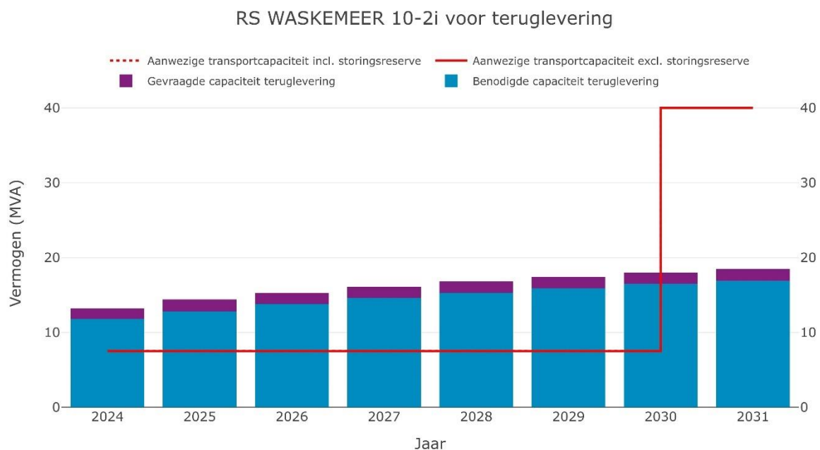
Figuur 3: Ontwikkeling van de aanwezig transportcapaciteit op congestiegebied Waskemeer tot en met het vierde kwartaal van 2030
