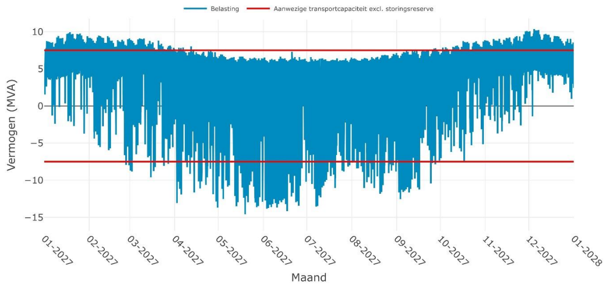
Verwachte belasting op RS WASKEMEER 10-2i voor het jaar 2027
