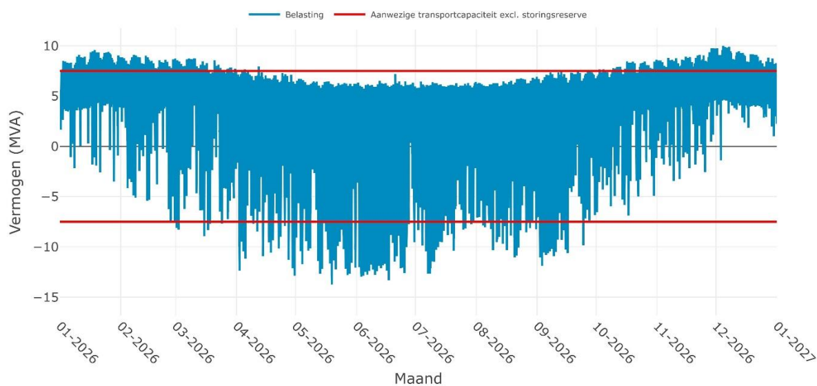
Verwachte belasting op RS WASKEMEER 10-2i voor het jaar 2026
