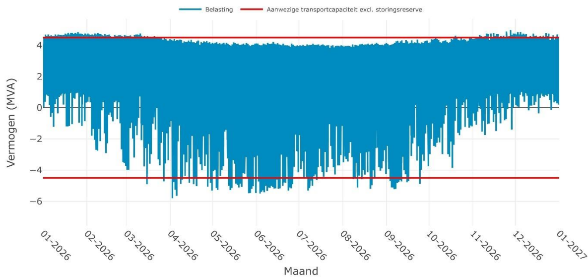
Verwachte belasting op SS OLDEBERKOOP 10-1i voor het jaar 2026
