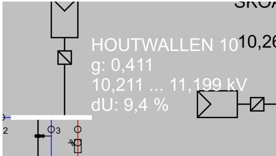
Figuur 5: Locatie met slechtste spanningsresultaten welke buiten de beleidsgrenzen vallen
