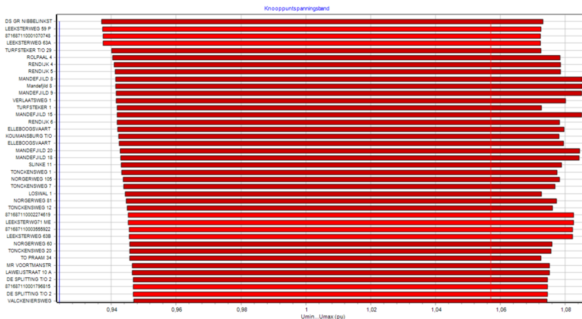
Figuur 2: Spanningscongestie
