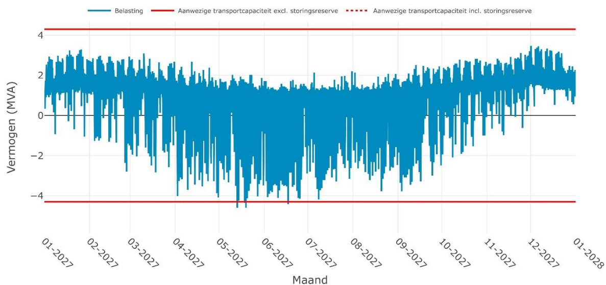
Verwachte belasting op SS HAULERWIJK 10-2i voor het jaar 2027
