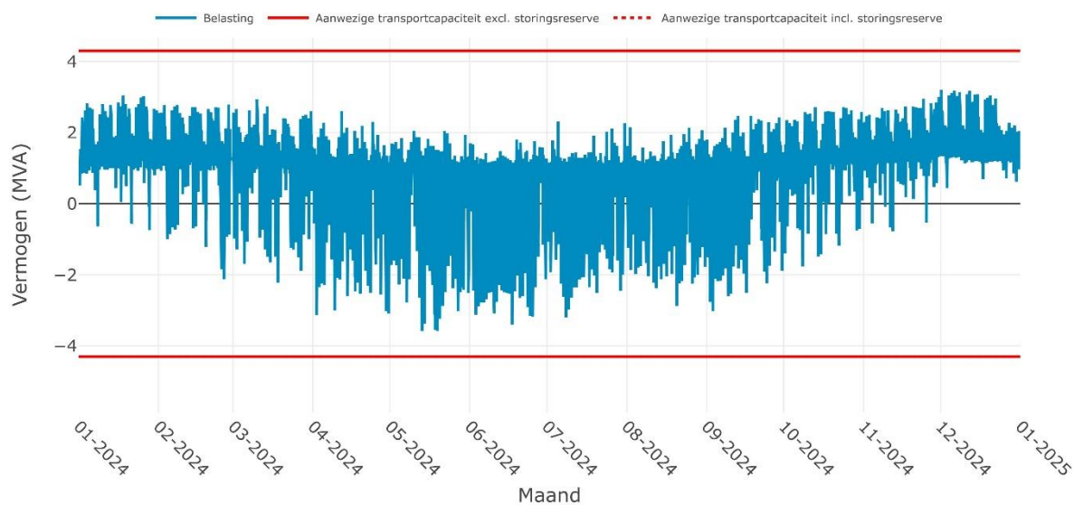
Verwachte belasting op SS HAULERWIJK 10-2i voor het jaar 2024
