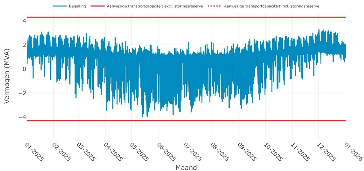
Verwachte belasting op SS HAULERWIJK 10-2i voor het jaar 2025
