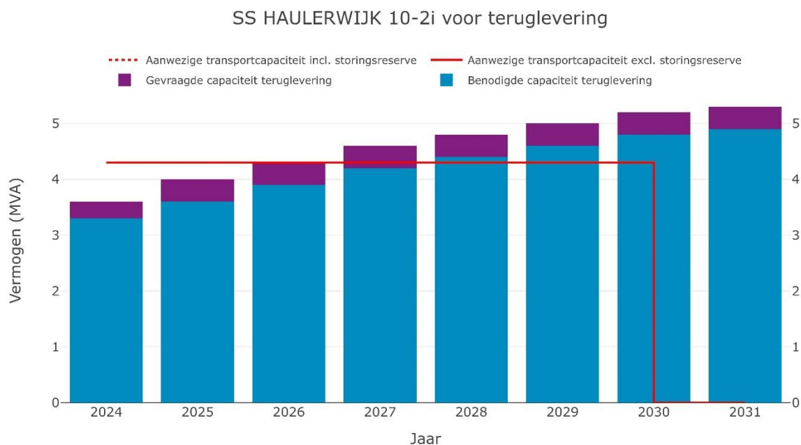
Figuur 3: Ontwikkeling van de aanwezig transportcapaciteit op Congestiegebied Haulerwijk tot en met het vierde kwartaal van 2030
