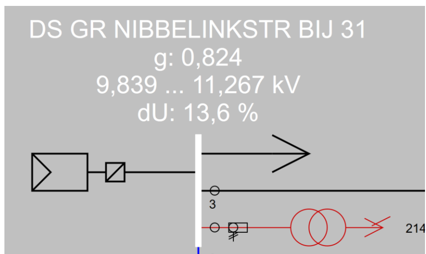
Figuur 4: Locatie met slechtste spanningsresultaten welke buiten de beleidsgrenzen vallen
