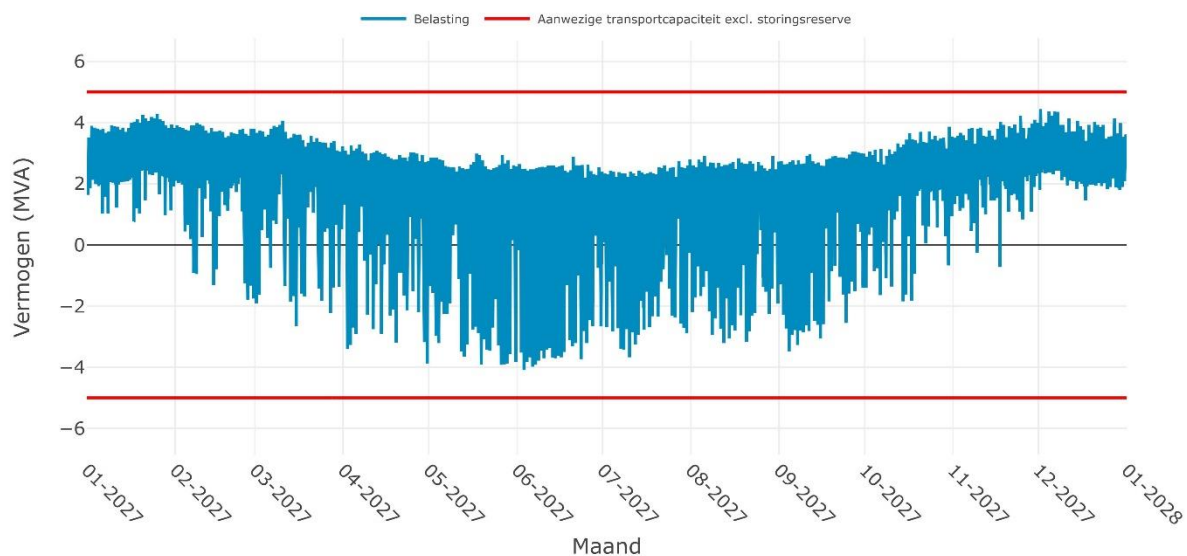
Verwachte belasting op SS APPELSCHA 10-2i voor het jaar 2027
