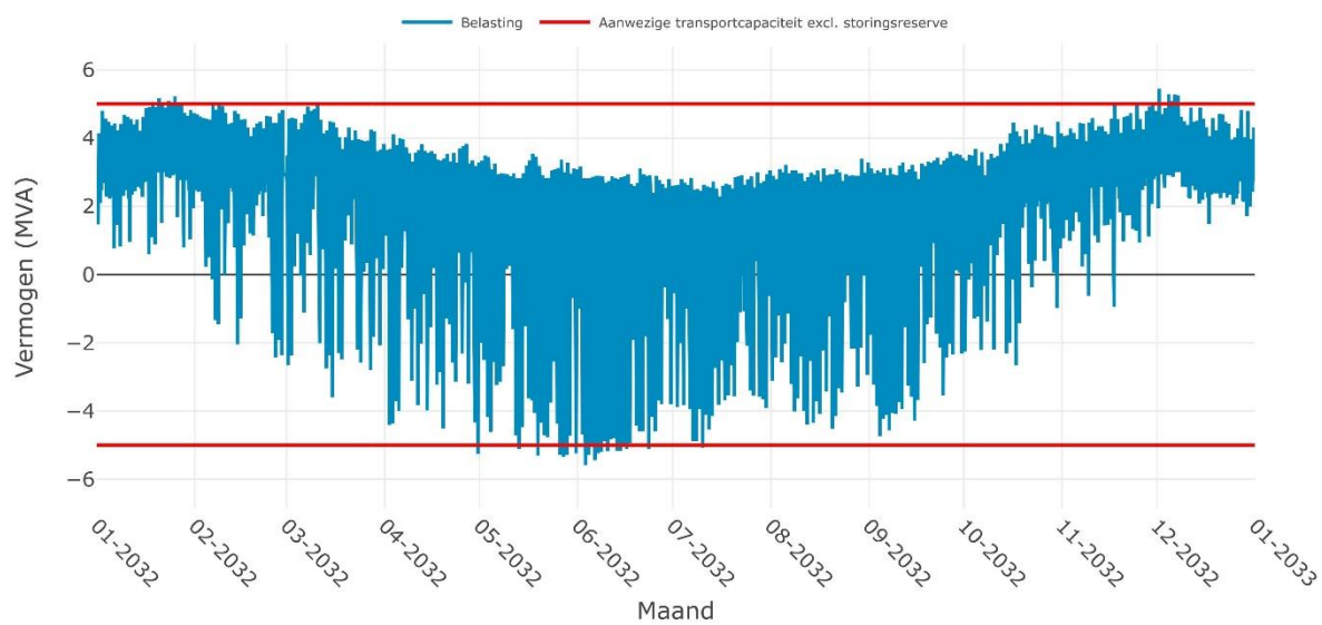
Verwachte belasting op SS APPELSCHA 10-2i voor het jaar 2032
