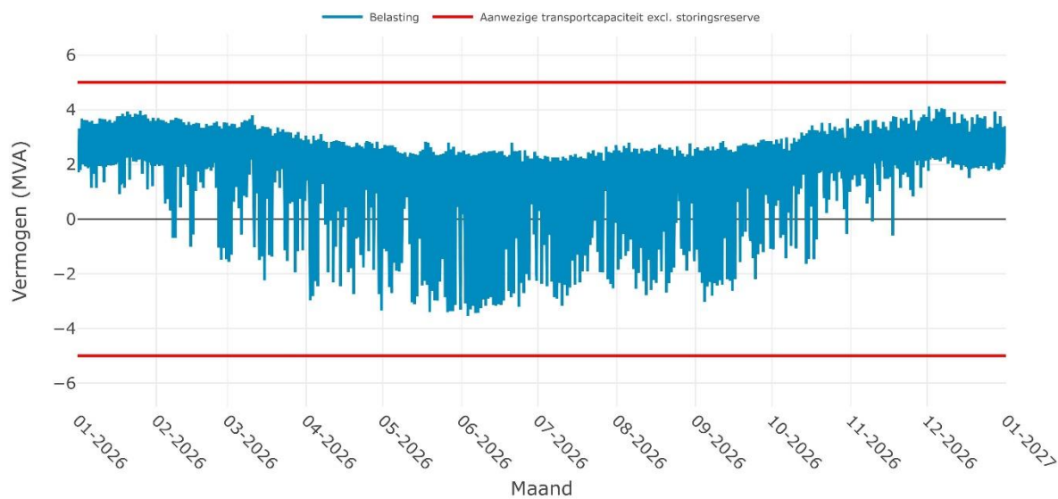
Verwachte belasting op SS APPELSCHA 10-2i voor het jaar 2026
