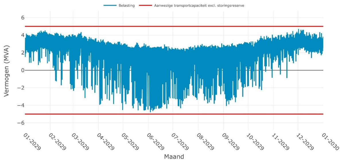
Verwachte belasting op SS APPELSCHA 10-2i voor het jaar 2029
