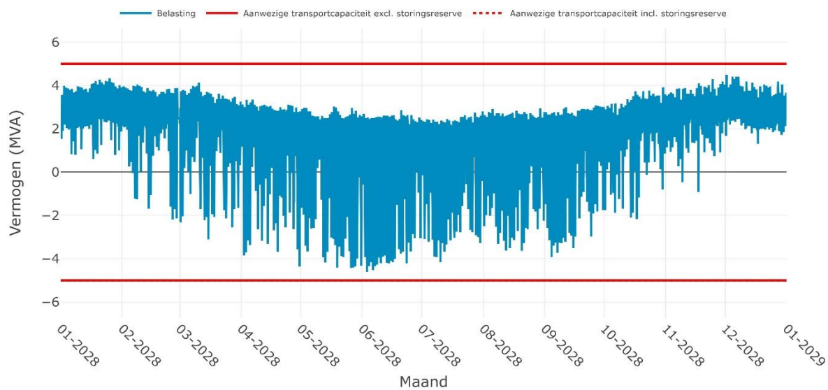
Verwachte belasting op SS APPELSCHA 10-2i voor het jaar 2028
