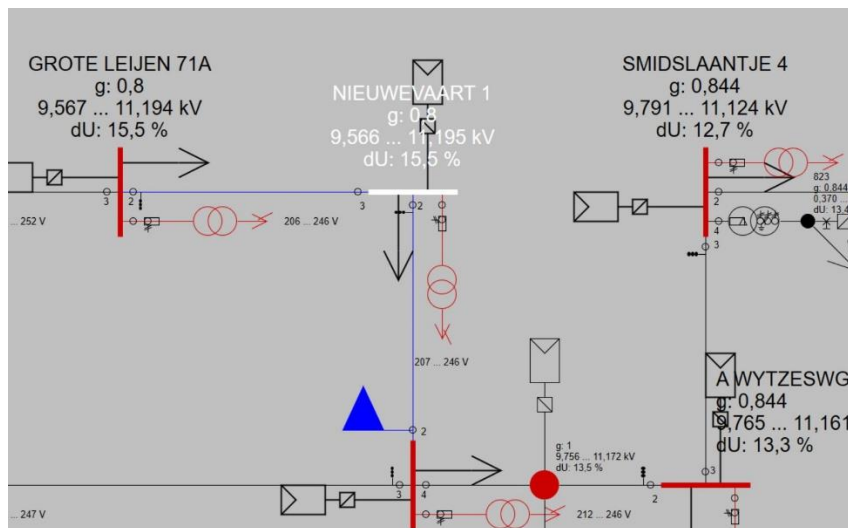
Figuur 5: Locatie met slechtste spanningsresultaten welke buiten de beleidsgrenzen vallen
