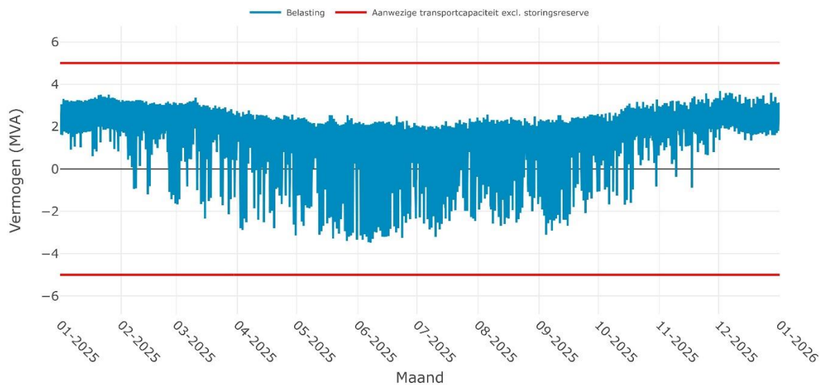
Verwachte belasting op SS APPELSCHA 10-2i voor het jaar 2025
