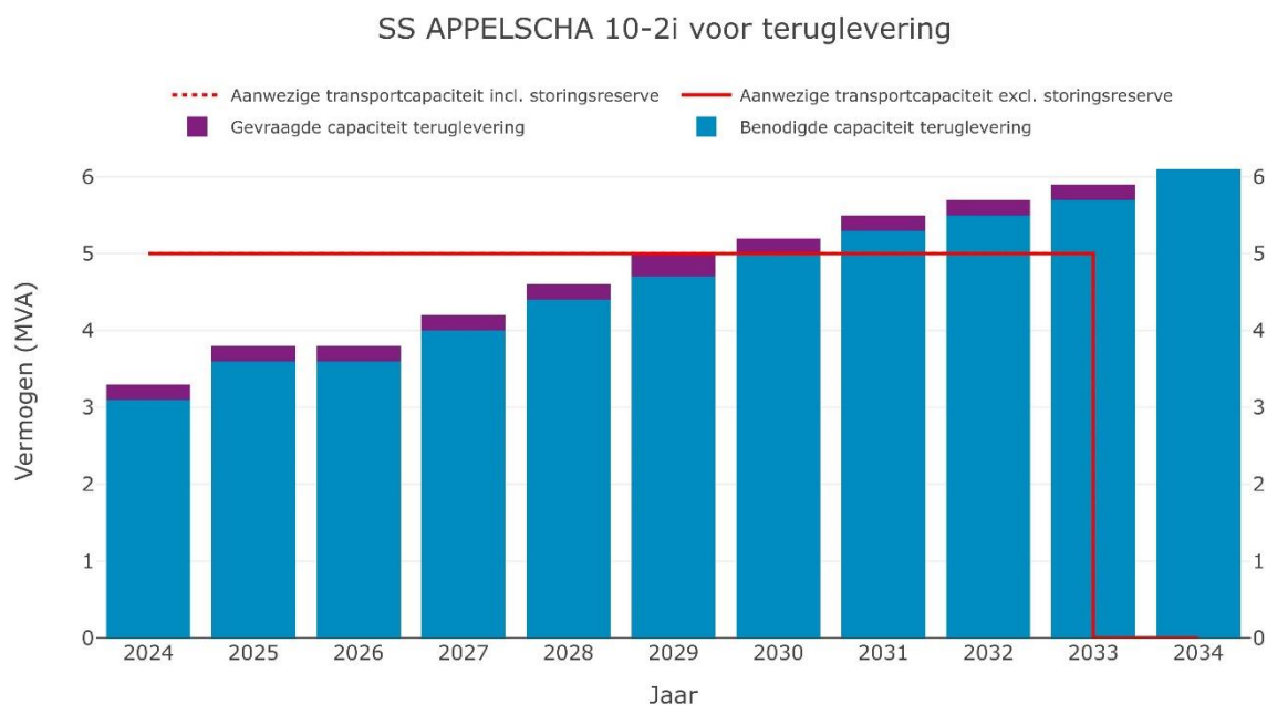
Figuur 2: Ontwikkeling van de aanwezige transportcapaciteit op congestiegebied Appelscha tot en met het vierde kwartaal van 2033
