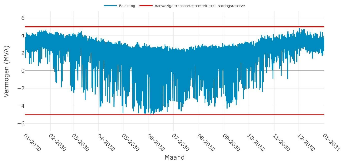
Verwachte belasting op SS APPELSCHA 10-2i voor het jaar 2030
