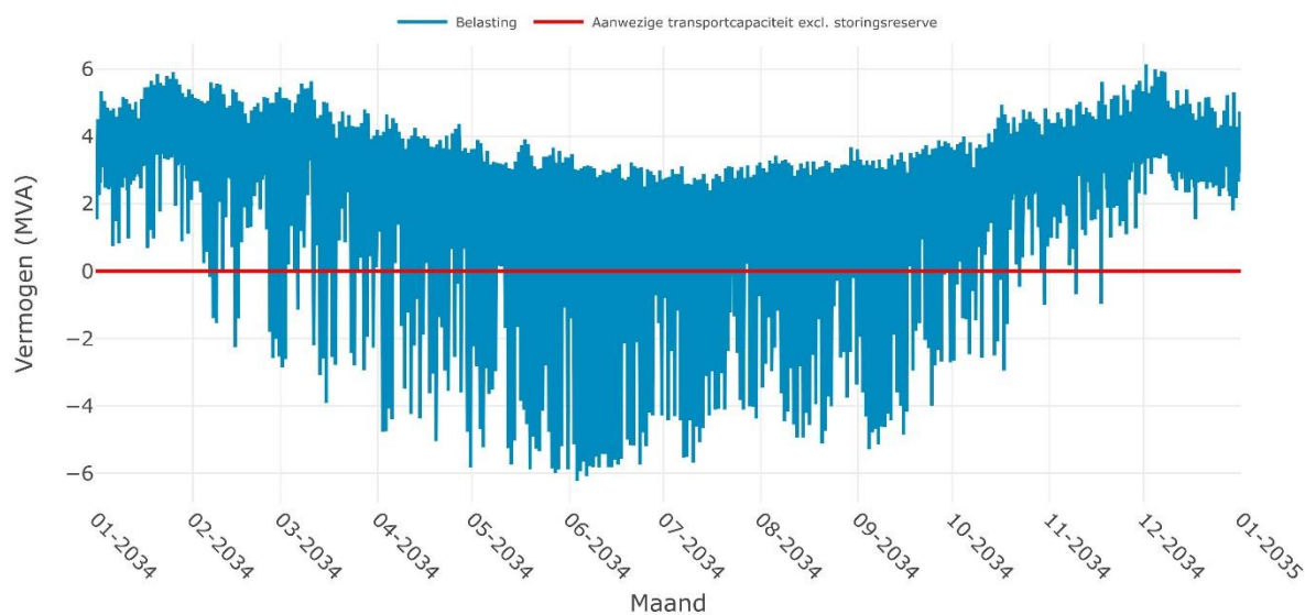
Verwachte belasting op SS APPELSCHA 10-2i voor het jaar 2034
