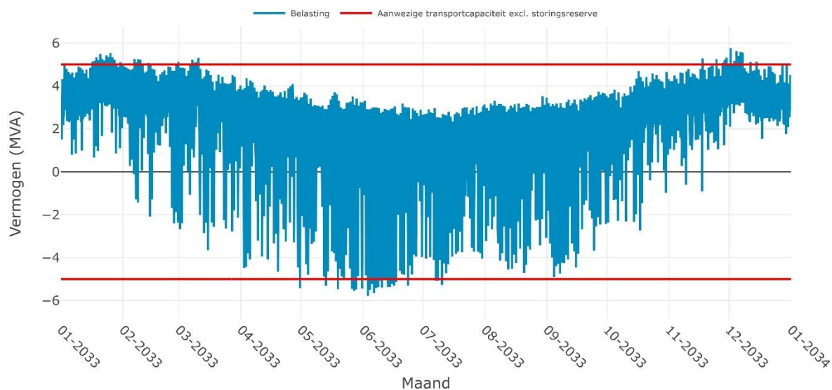
Verwachte belasting op SS APPELSCHA 10-2i voor het jaar 2033
