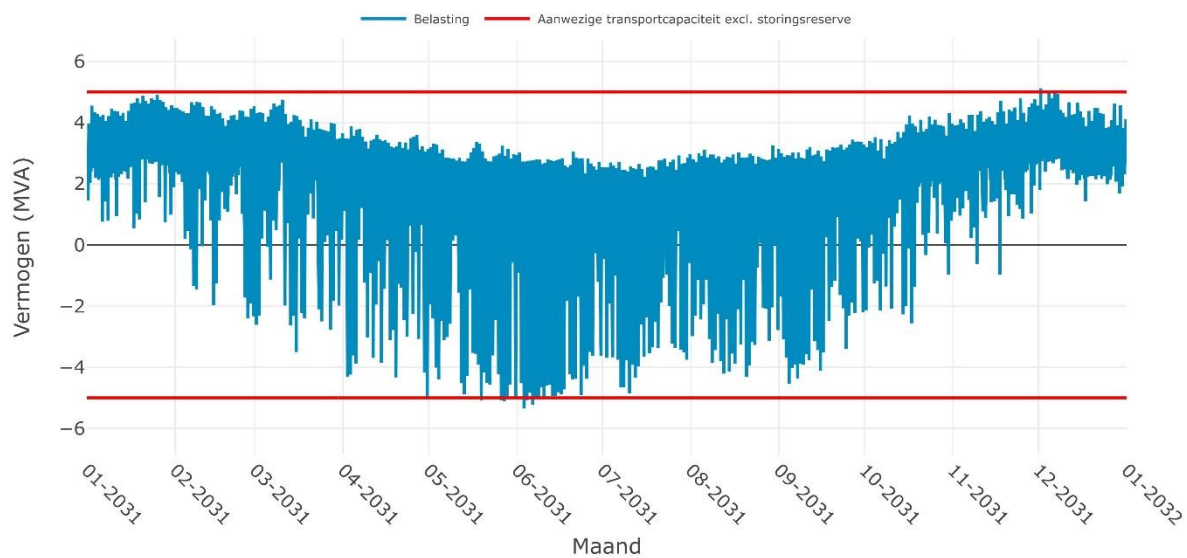
Verwachte belasting op SS APPELSCHA 10-2i voor het jaar 2031
