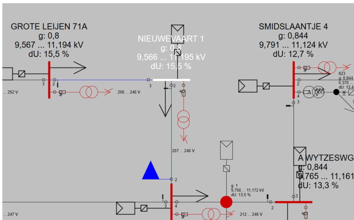
Figuur 5: Locatie met de slechtste spanning resultaten welke buiten de beleidsgrenzen vallen
