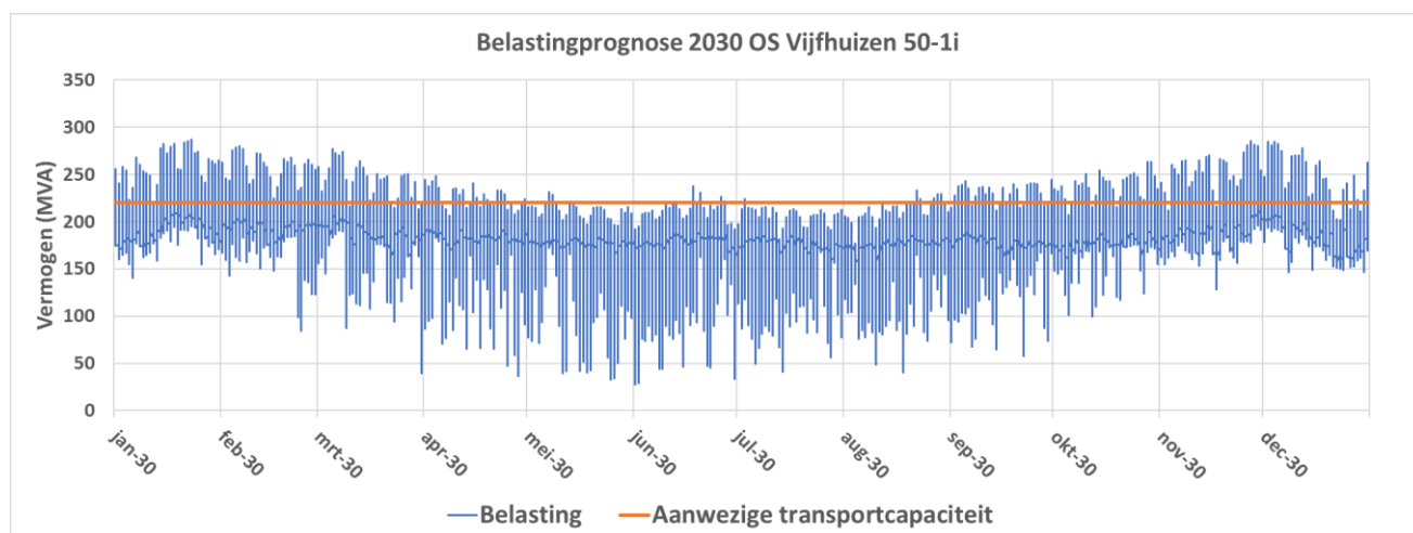
Figuur 3: Verwachte belasting op de kritieke netcomponent in het laatste jaar van de verwachte congestie.
