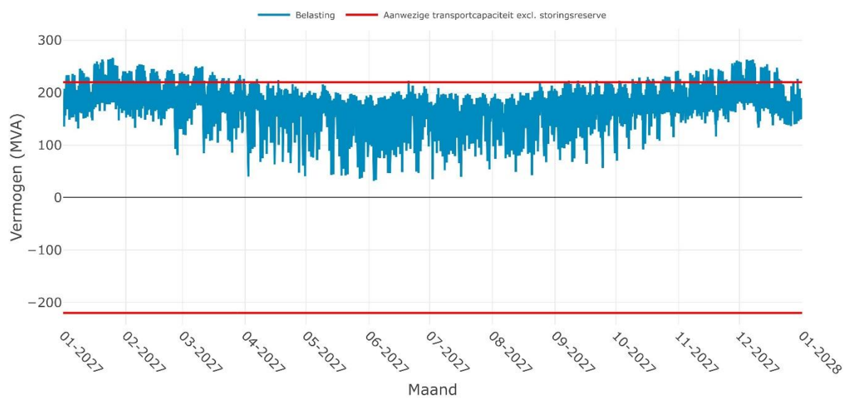
Verwachte belasting op OS VIJFHUIZEN 50-1i voor het jaar 2027
