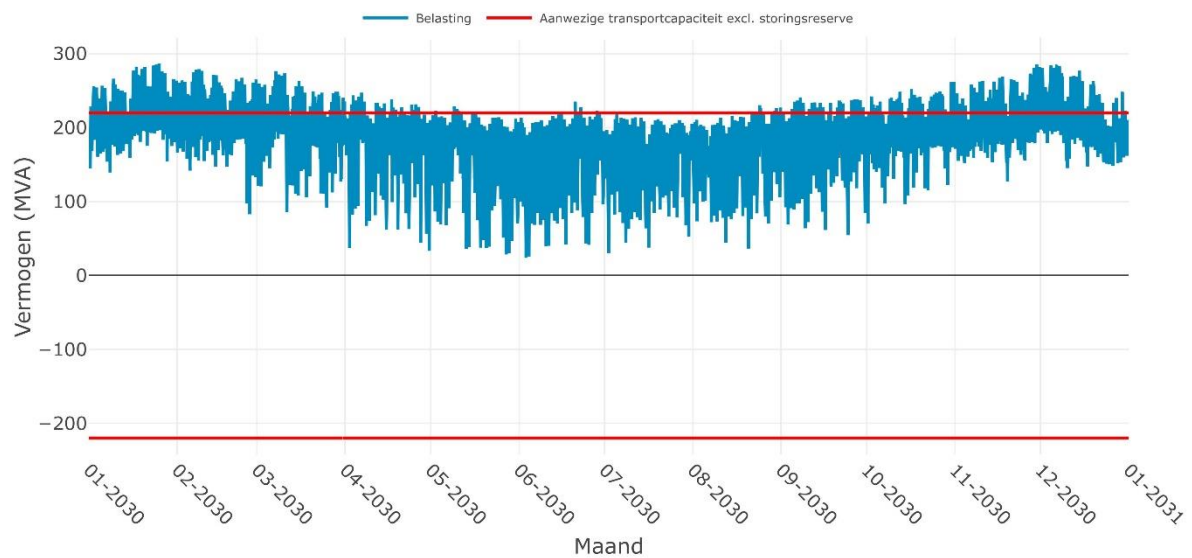
Verwachte belasting op OS VIJFHUIZEN 50-1i voor het jaar 2030
