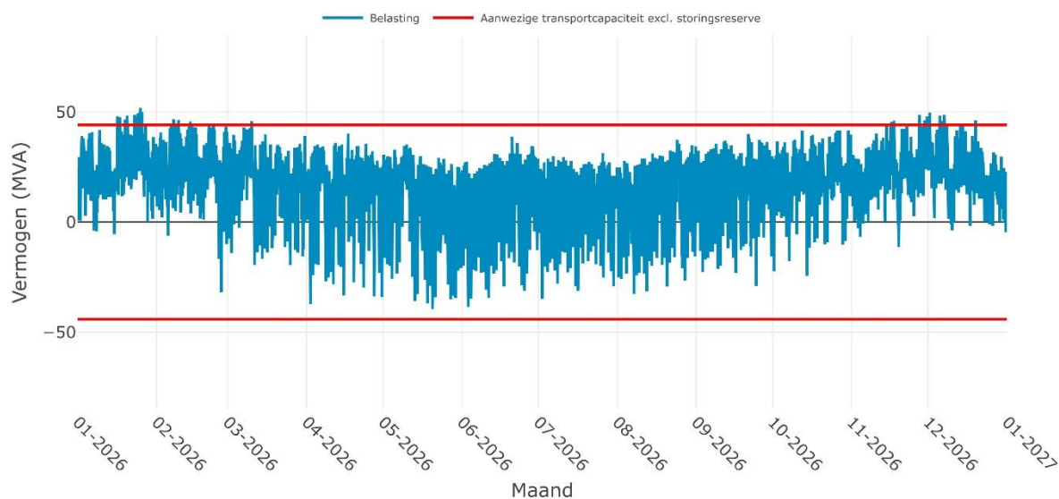
Verwachte belasting op OS CULEMBORG 10-1i voor het jaar 2026
