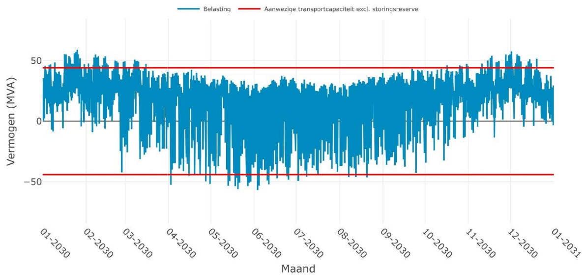
Verwachte belasting op OS CULEMBORG 10-1i voor het jaar 2030
