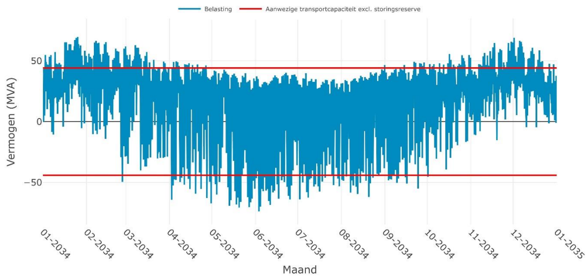
Verwachte belasting op OS CULEMBORG 10-1i voor het jaar 2034
