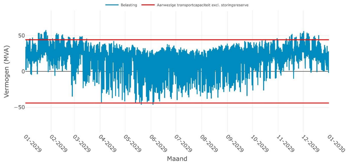
Verwachte belasting op OS CULEMBORG 10-1i voor het jaar 2029
