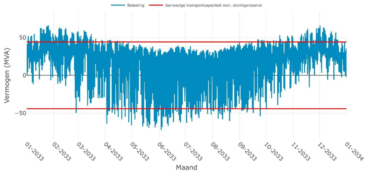
Verwachte belasting op OS CULEMBORG 10-1i voor het jaar 2033
