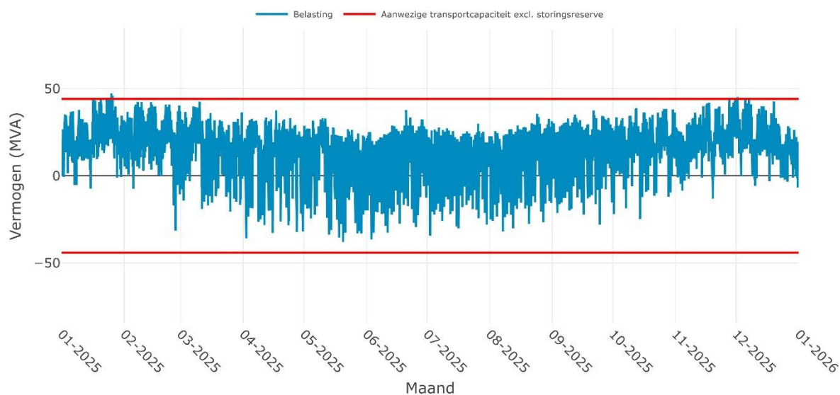
Verwachte belasting op OS CULEMBORG 10-1i voor het jaar 2025
