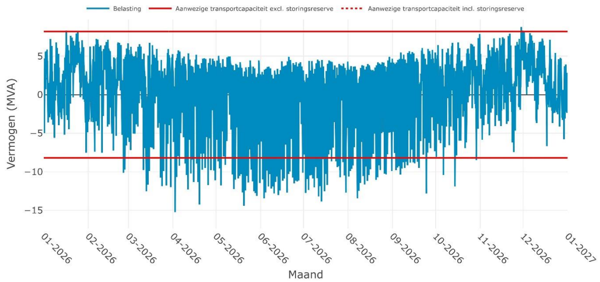
Verwachte belasting op RS HALLUM 10-1i voor het jaar 2026
