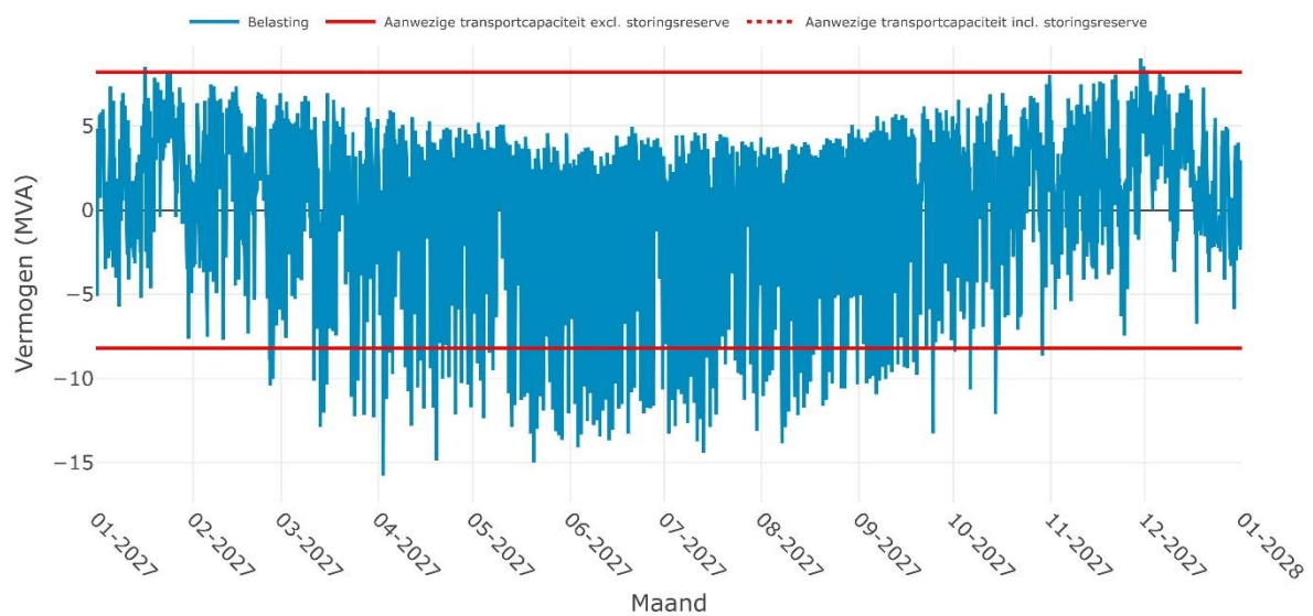
Verwachte belasting op RS HALLUM 10-1i voor het jaar 2027
