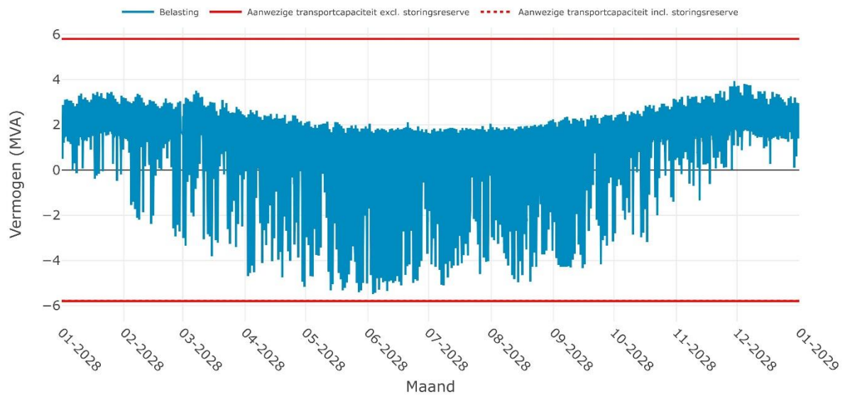
Verwachte belasting op SS NOORDBERGUM 10-2i voor het jaar 2028
