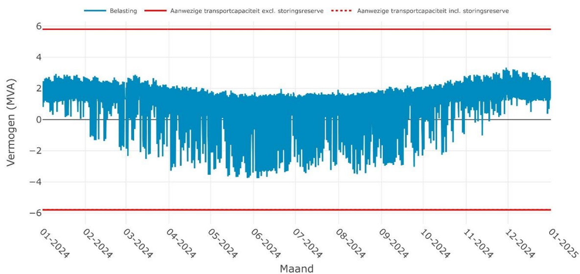
Verwachte belasting op SS NOORDBERGUM 10-2i voor het jaar 2024
