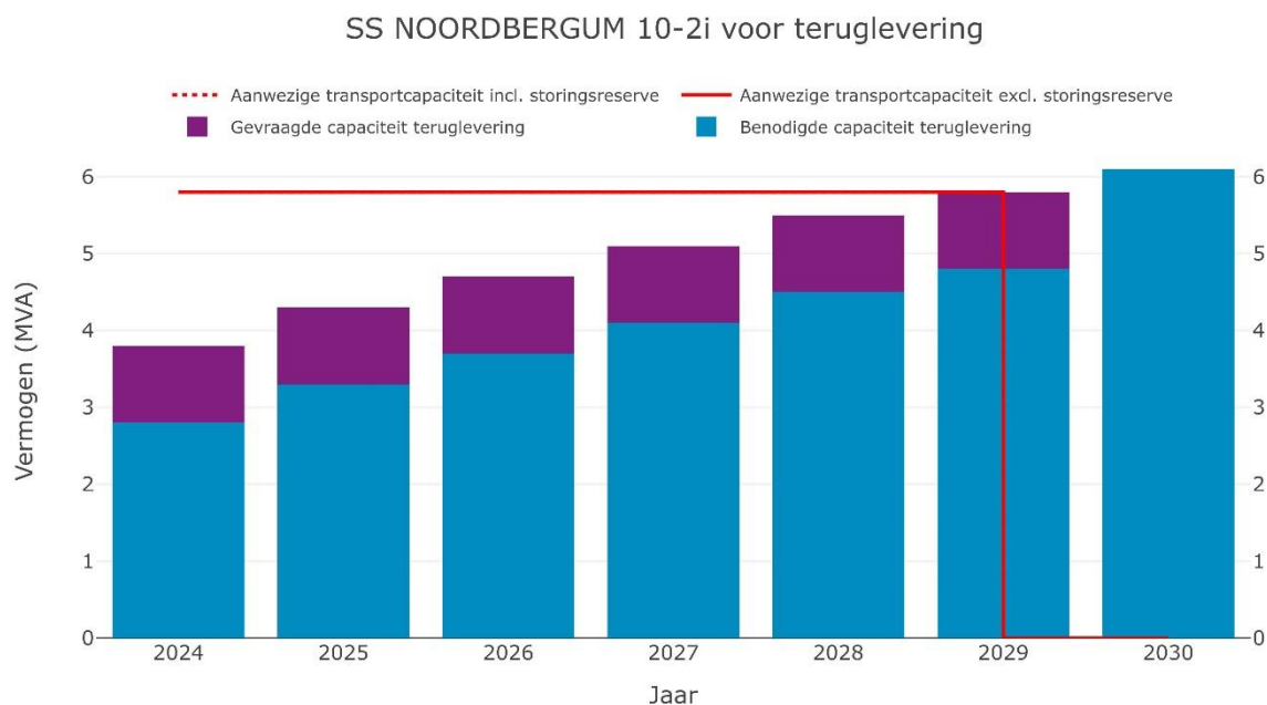
Figuur 3: Ontwikkeling van de aanwezig transportcapaciteit op congestiegebied Noordbergum tot en met het tweede kwartaal van 2029
