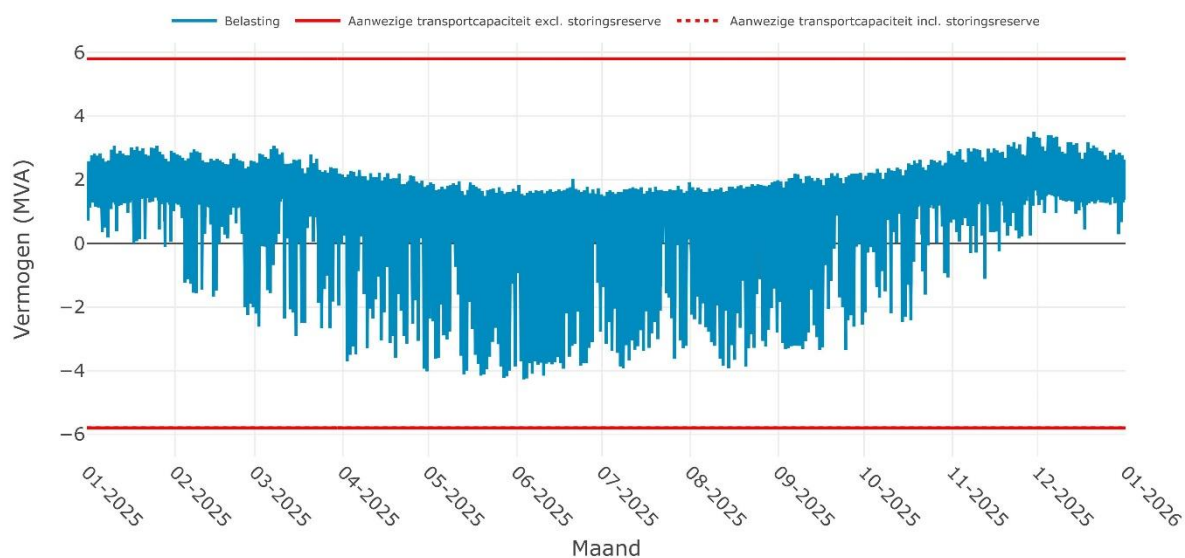
Verwachte belasting op SS NOORDBERGUM 10-2i voor het jaar 2025
