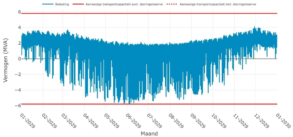
Verwachte belasting op SS NOORDBERGUM 10-2i voor het jaar 2029
