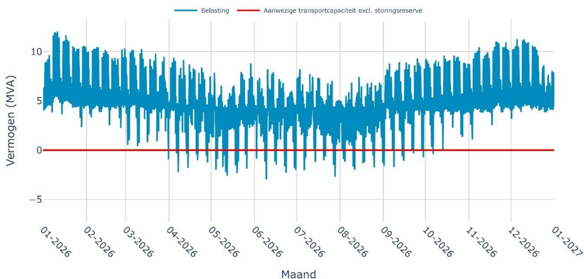
Verwachte belasting op SS Bisschopsrak 10-1i + 10-2i voor het jaar 2026
