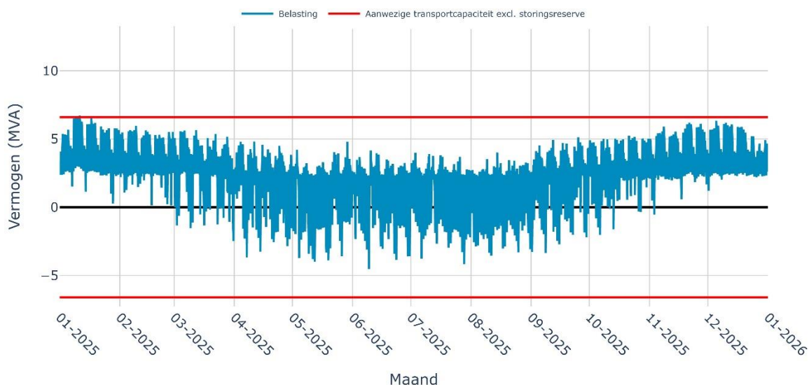
Verwachte belasting op SS Bisschopsrak 10-1i + 10-2i voor het jaar 2025
