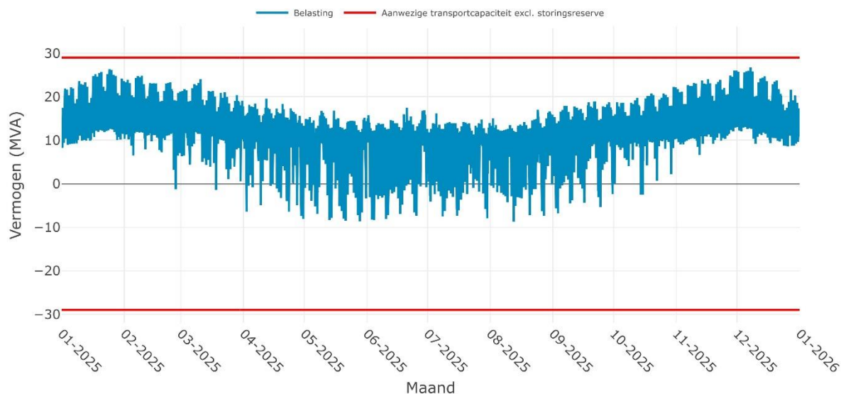
Verwachte belasting op OS SCHENKENSCHANS 10-2i voor het jaar 2025
