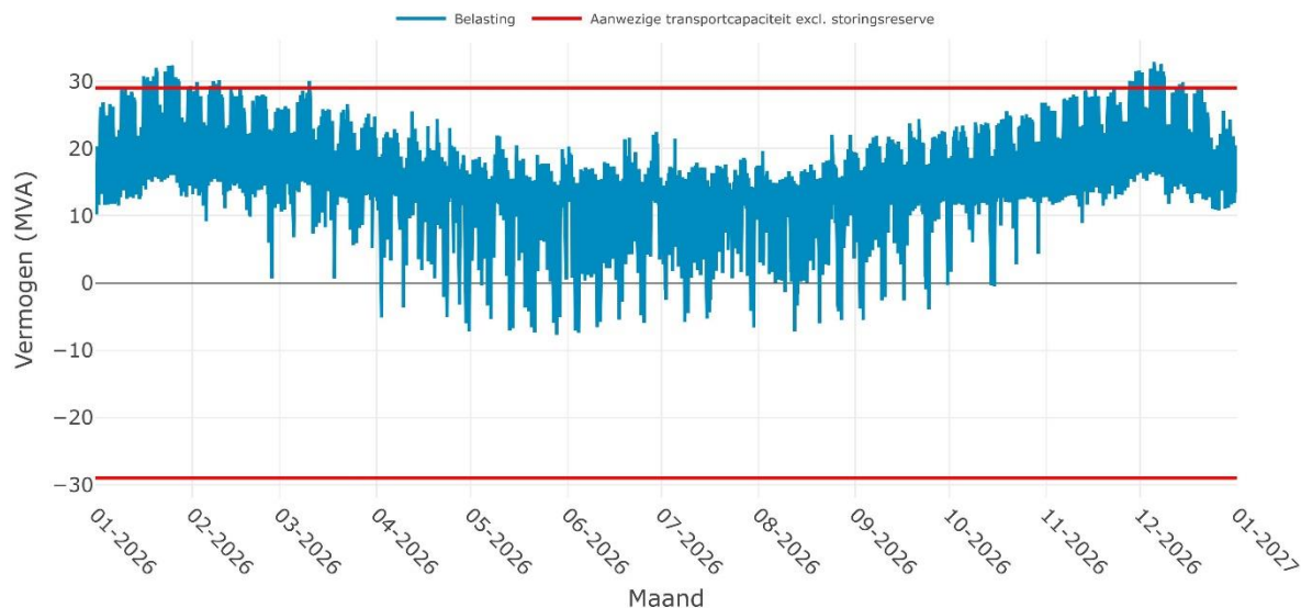
Verwachte belasting op OS SCHENKENSCHANS 10-2i voor het jaar 2026
