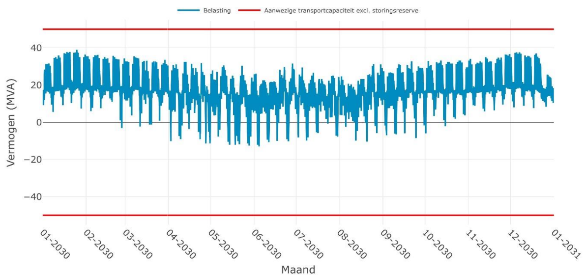
Verwachte belasting op OS FRANKENENG 10-1i voor het jaar 2030
