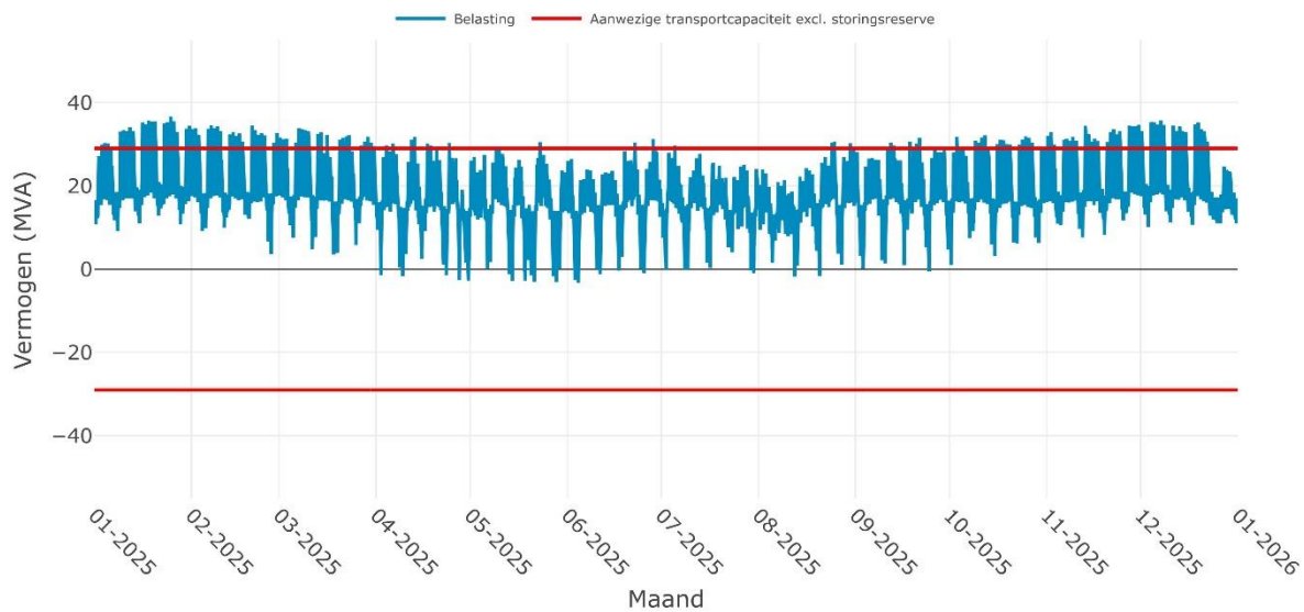
Verwachte belasting op OS FRANKENENG 10-1i voor het jaar 2025
