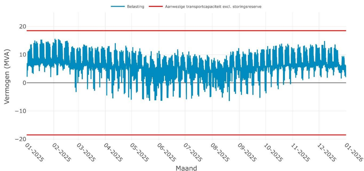
Verwachte belasting op RS RIJNWAARDEN 10-1i voor het jaar 2025
