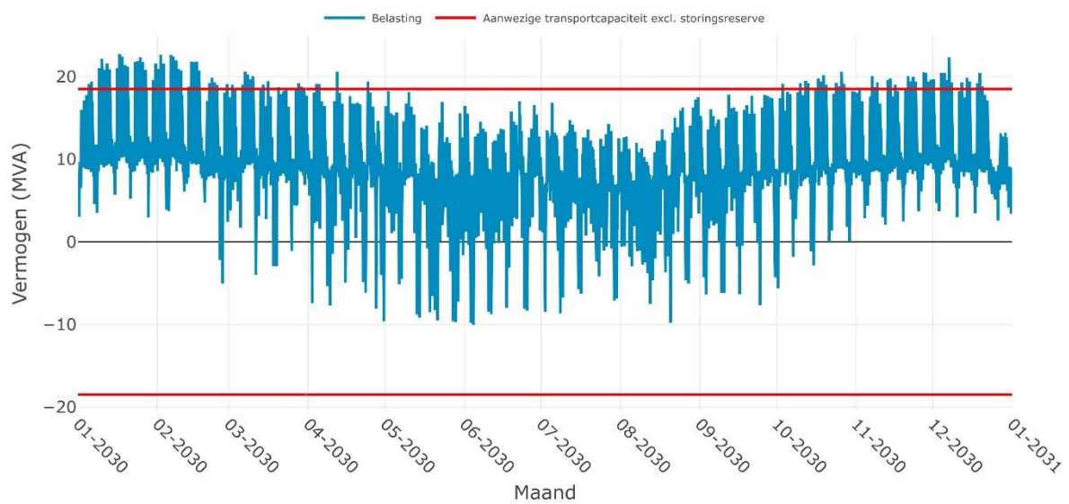
Verwachte belasting op RS RIJNWAARDEN 10-1i voor het jaar 2030
