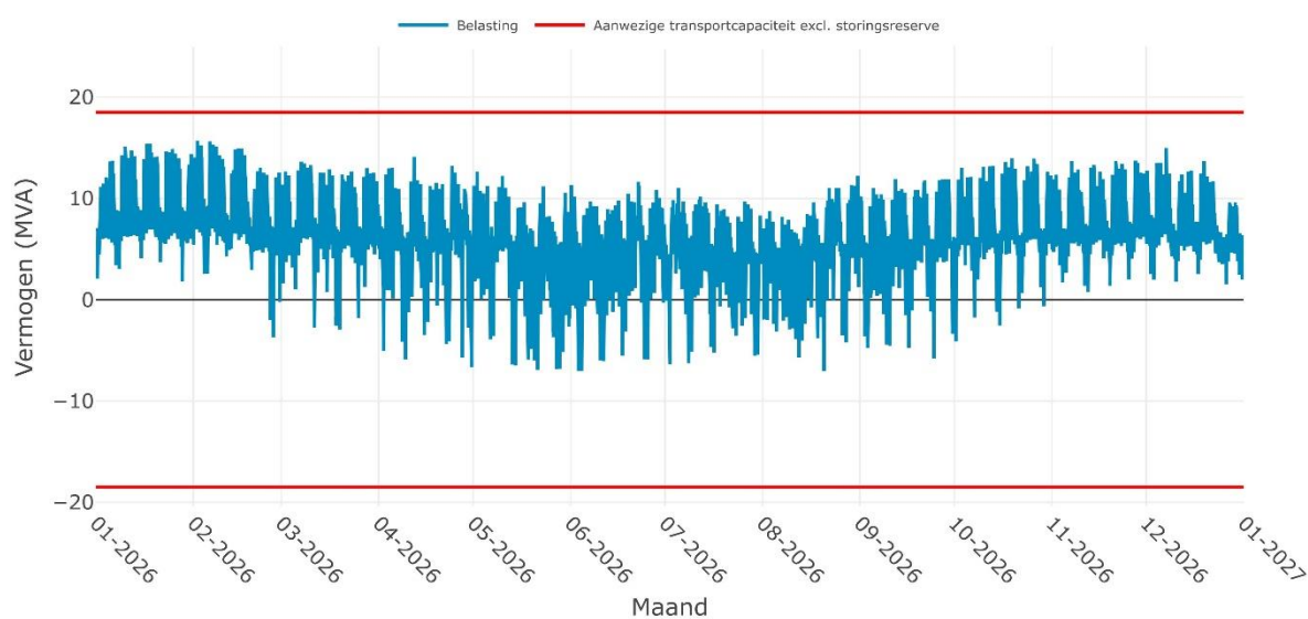
Verwachte belasting op RS RIJNWAARDEN 10-1i voor het jaar 2026
