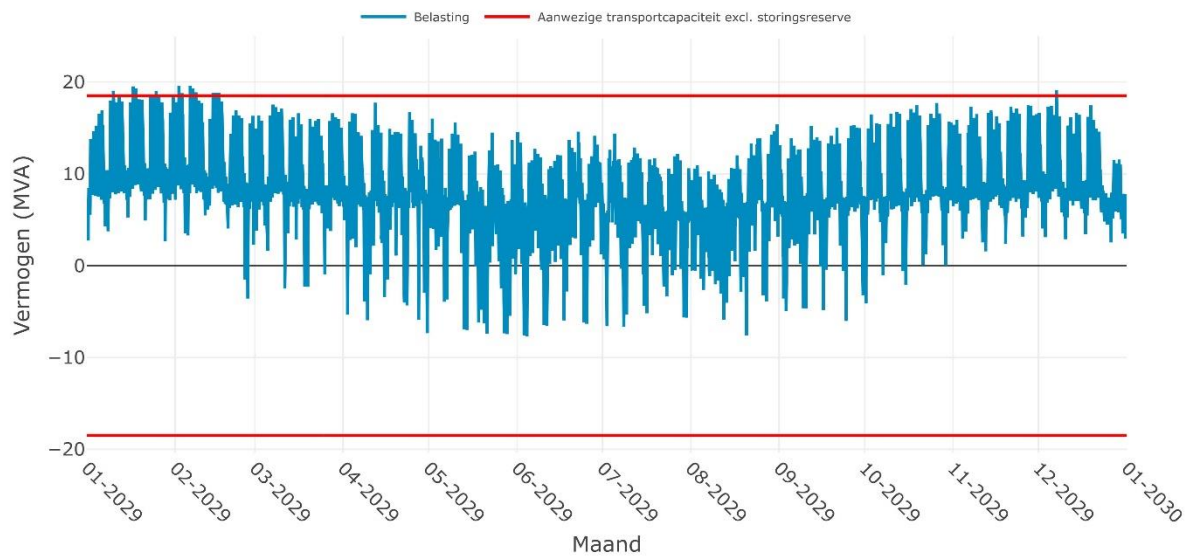
Verwachte belasting op RS RIJNWAARDEN 10-1i voor het jaar 2029
