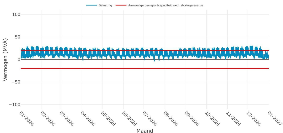
Verwachte belasting op SS ALKMAAR BOEKELERMEER 10-1i voor het jaar 2026
