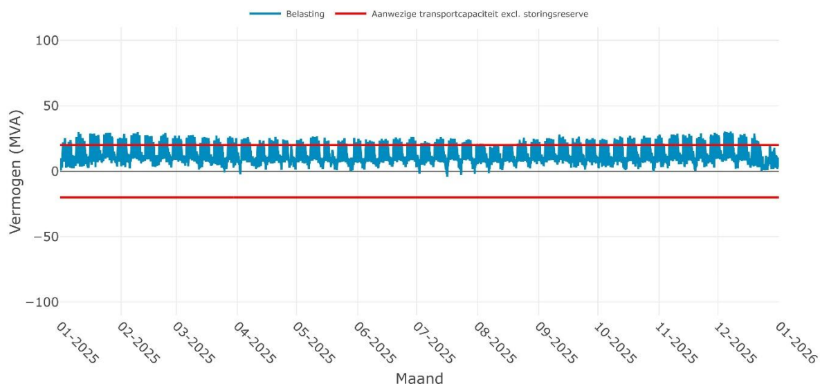
Verwachte belasting op SS ALKMAAR BOEKELERMEER 10-1i voor het jaar 2025
