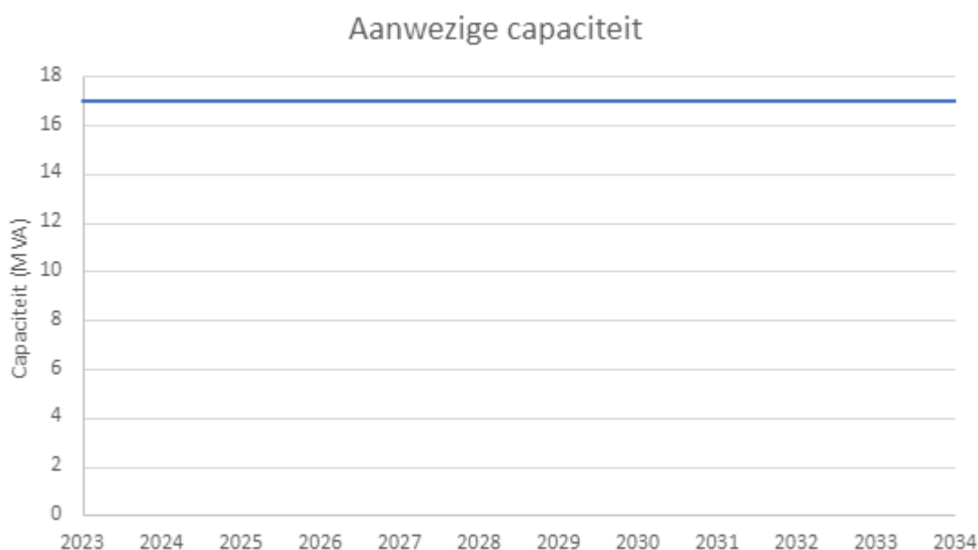
Figuur 2: Ontwikkeling van aanwezige transportcapaciteit op verdeelstation Alkmaar Boekelermeer.
