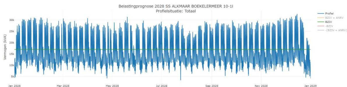
Figuur 3: Verwachte belasting op de kritieke netcomponent in het zwaarste jaar van de verwachte congestie.
