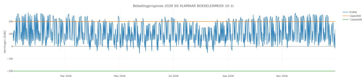
Figuur 5: Verwachte belasting in het laatste jaar van de verwachte congestie bij verdeelstation Alkmaar Boekelermeer.
