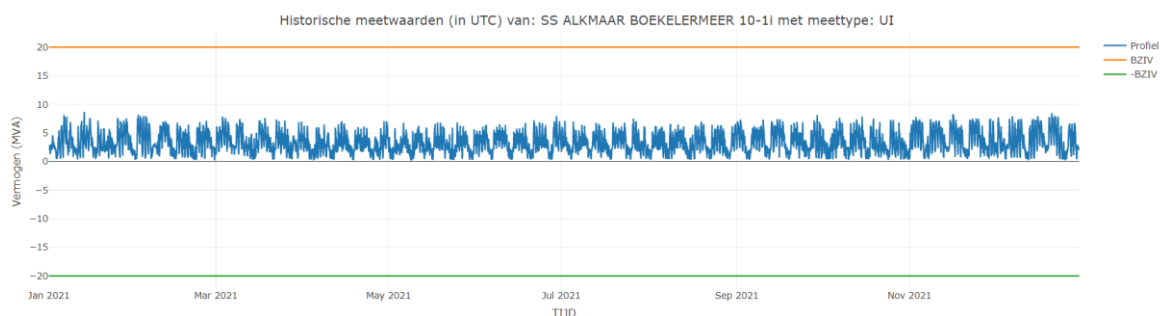
Figuur 4: Gerealiseerde vermogenscurve in het afgelopen jaar bij verdeelstation Alkmaar Boekelermeer.
