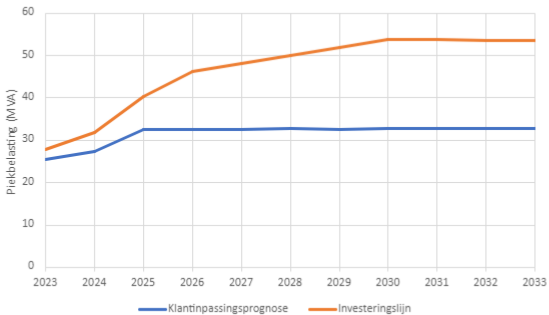
Figuur 4: Verwachte piekbelasting op verdeelstation Alkmaar Boekelermeer per jaar tot en met begin 2030.
