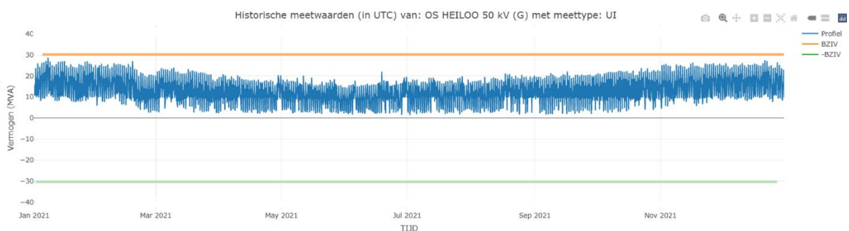
Figuur 5: Gerealiseerde vermogenscurve in het afgelopen jaar bij verdeelstation Heiloo.
