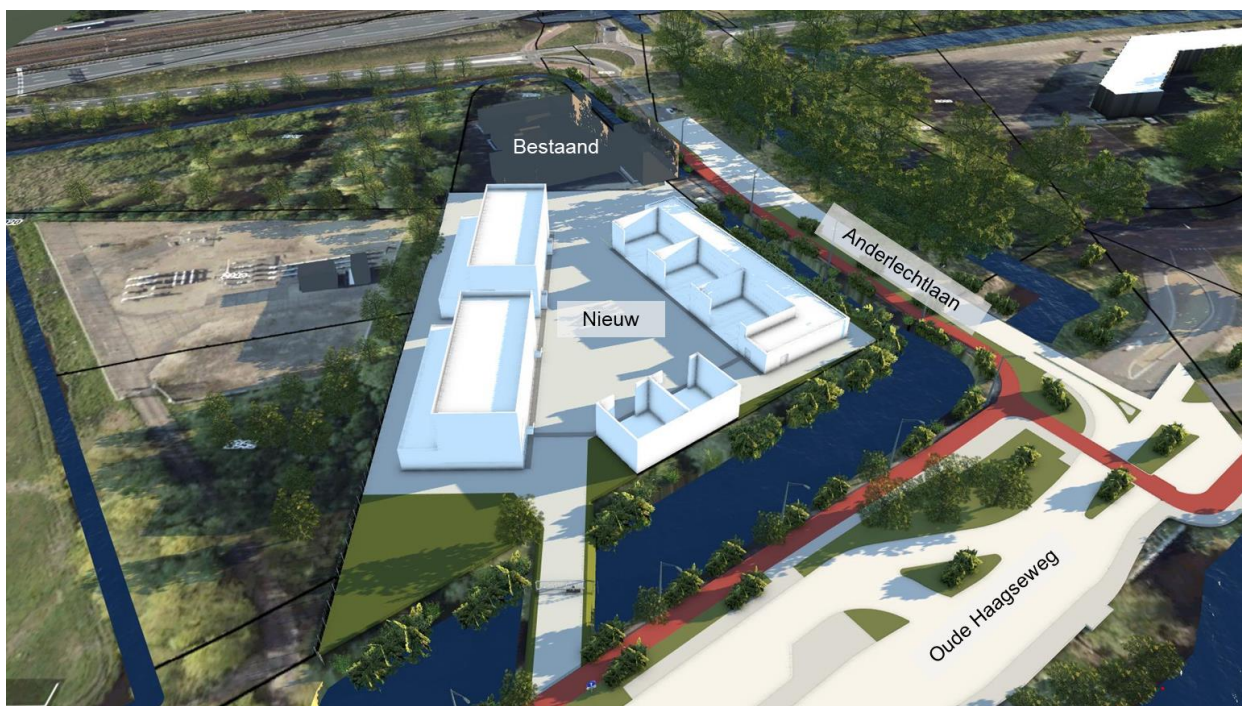
Het nieuwe elektriciteitsstation komt ten zuiden van het bestaande elektriciteitsstation. Op deze afbeelding ziet u waar de gebouwen komen te staan. De architect maakt een ontwerp voor het uiterlijk van het elektriciteitsstation.
