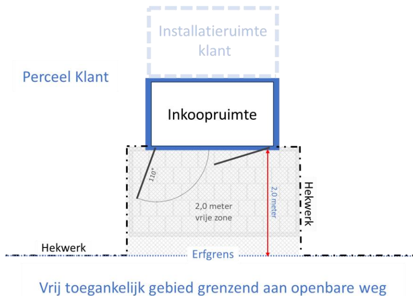
Figuur 4 Schematische weergave van een inkoopruimte, inclusief obstakelvrije zone, gesitueerd aan de erfgrans.
