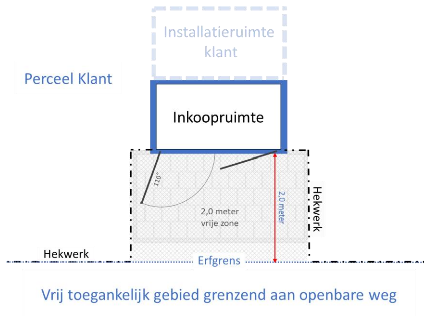
Figuur 4 Schematische weergave van een inkoopruimte, inclusief obstakelvrije zone, gesitueerd aan de erfgrans.
