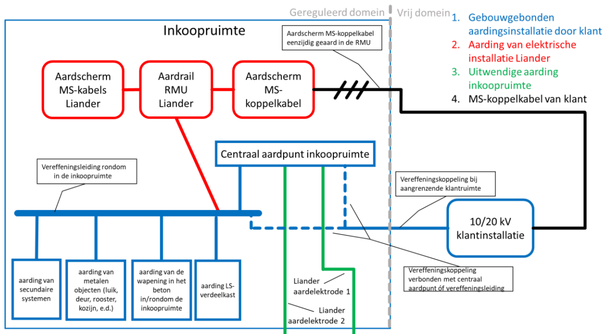
Figuur 6 Schematisch overzicht van aardingsinstallatie in en rondom de inkoopruimte
