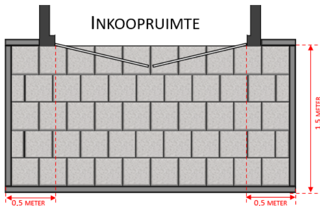
Figuur 5 Schematische weergave afmetingen straatwerk voor de toegangsdeur(en) van een inkoopruimte
