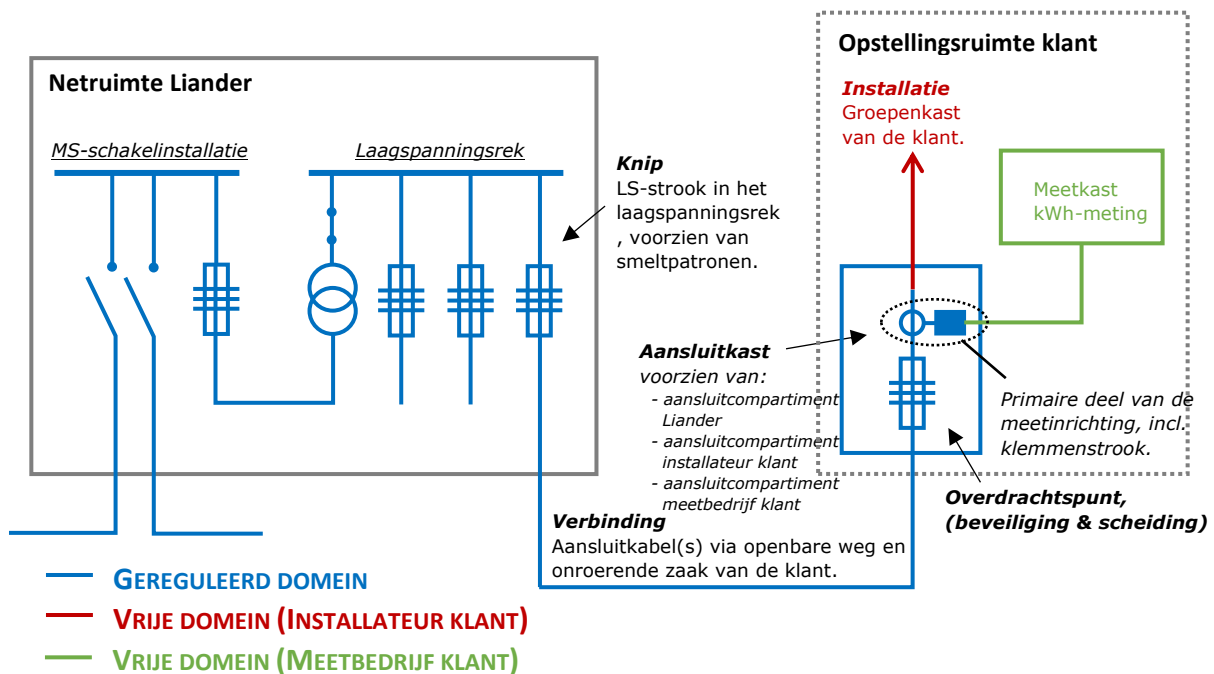
Figuur 3 Schematische weergave aansluitmethode AC4 klantaansluiting, opbouw conform Tarievenscode Elektriciteit, inclusief demarcatie gereguleerd en vrij domein.
