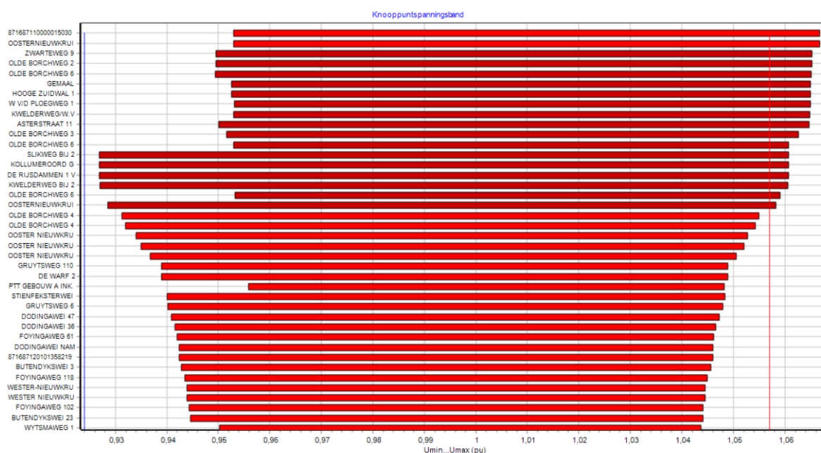
Figuur 2: Spanningscongestie
