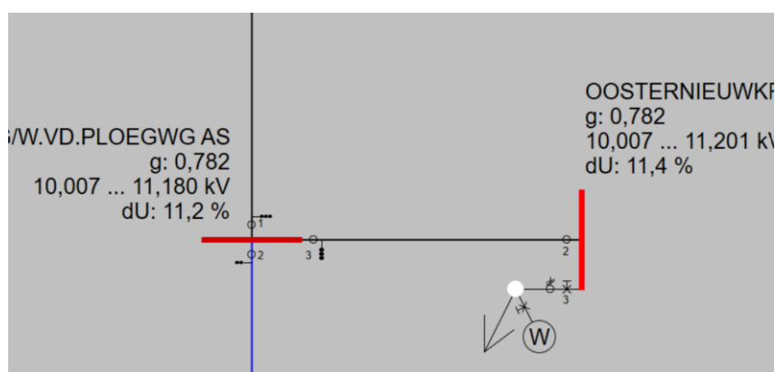
Figuur 4: Locatie met slechtste spanningsresultaten welke buiten de beleidsgrenzen vallen
